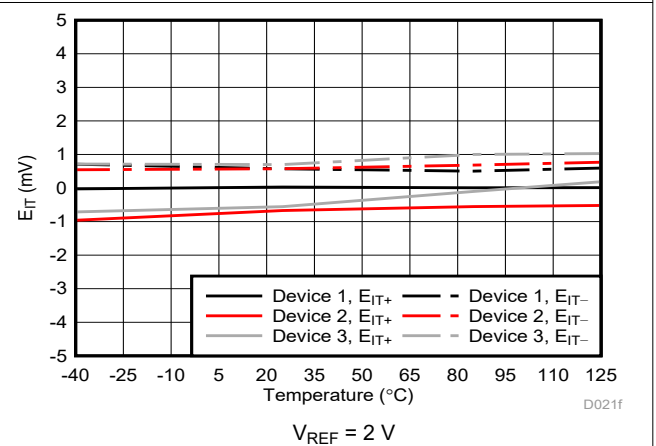
图 6-20. 跳变阈值误差与温度间的关系
