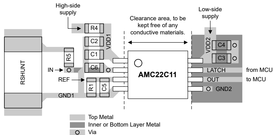
图 8-5. 建议布局 AMC22C11
