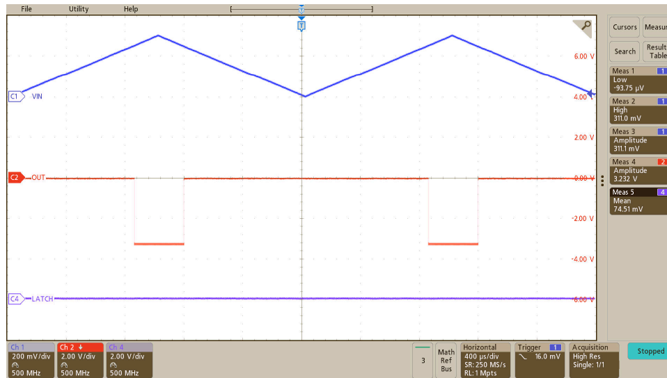
图 8-2. AMC22C11 对三角输入波形的输出响应
