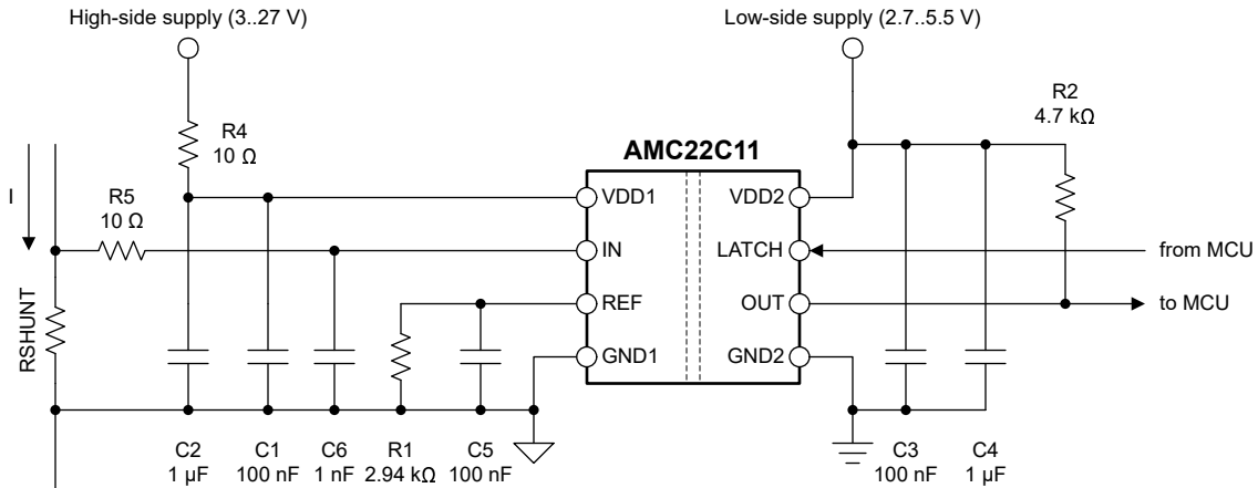
图 8-4. 去耦 AMC22C11
