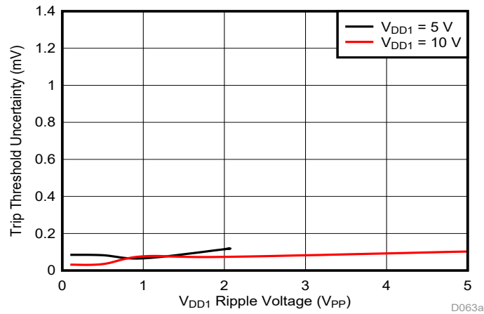
图 8-3. 跳变阈值对 V_{\text{DD1}} 纹波电压的灵敏度 ( f_{\text{RIPPLE}} = 10\text{kHz} )
