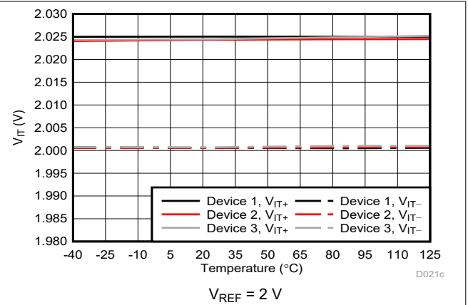
图 6-18. 跳变阈值与温度间的关系
