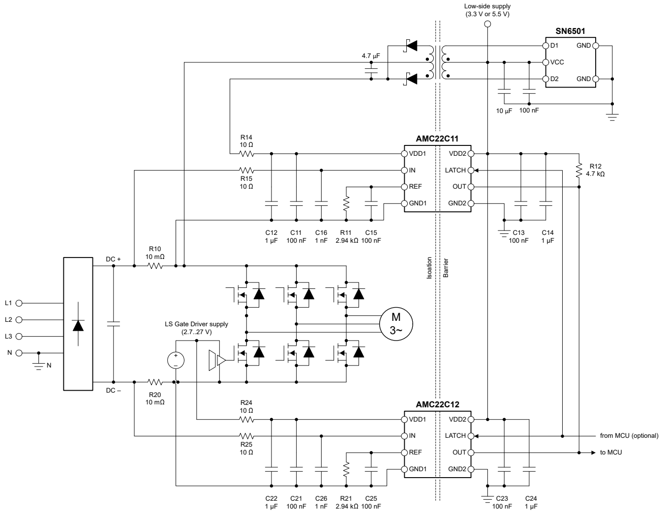
图 8-1. 使用 AMC22C11 进行 DC+ 过流检测
