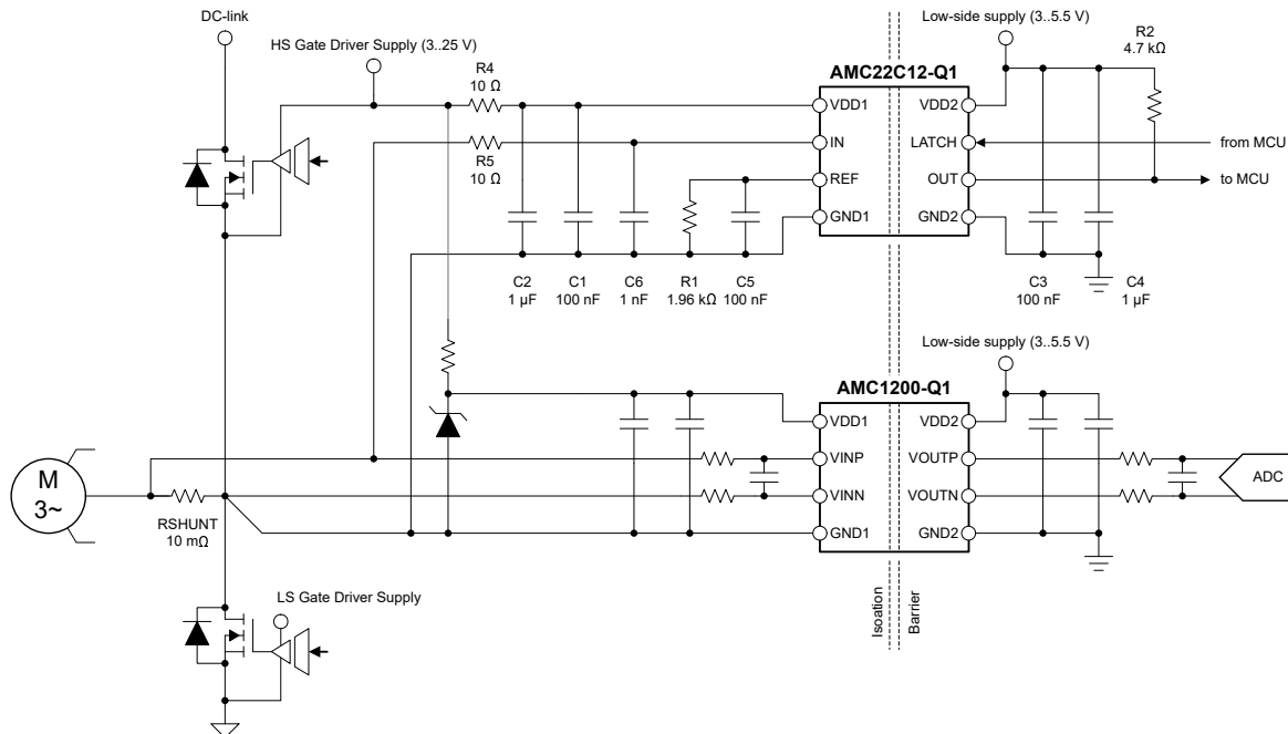
图 8-1. 使用 AMC22C12-Q1 进行过流检测
