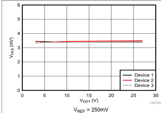
图 6-15. Cmp0 跳变阈值迟滞与电源电压间的关系
