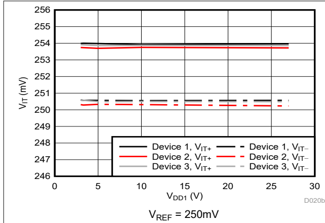
图 6-11. Cmp0 跳变阈值与电源电压间的关系
