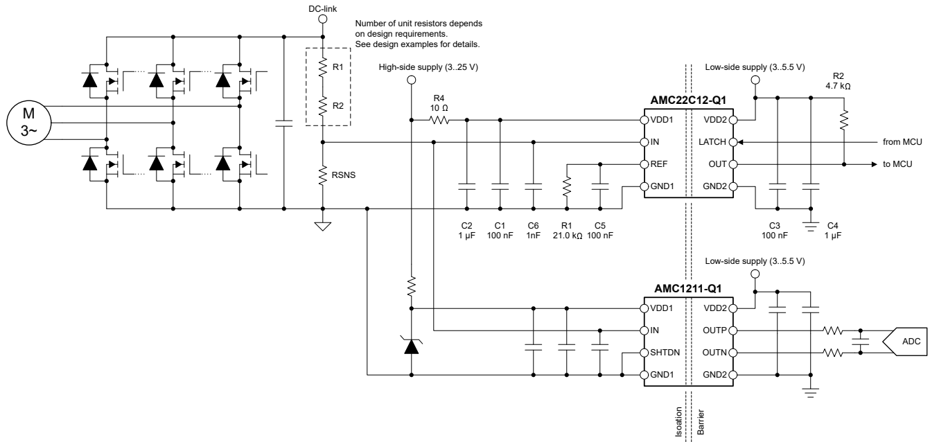
图 8-2. 使用 AMC22C12-Q1 进行过压检测
