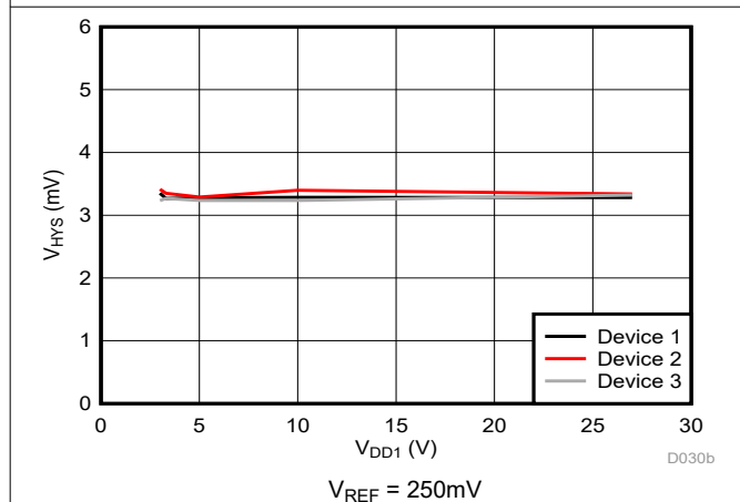
图 6-33. Cmp1 跳变阈值迟滞与电源电压间的关系
