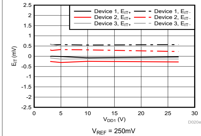
图 6-13. Cmp0 跳变阈值误差与电源电压间的关系
