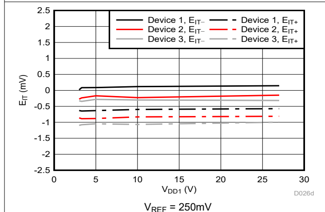
图 6-31. Cmp1 跳变阈值误差与电源电压间的关系
