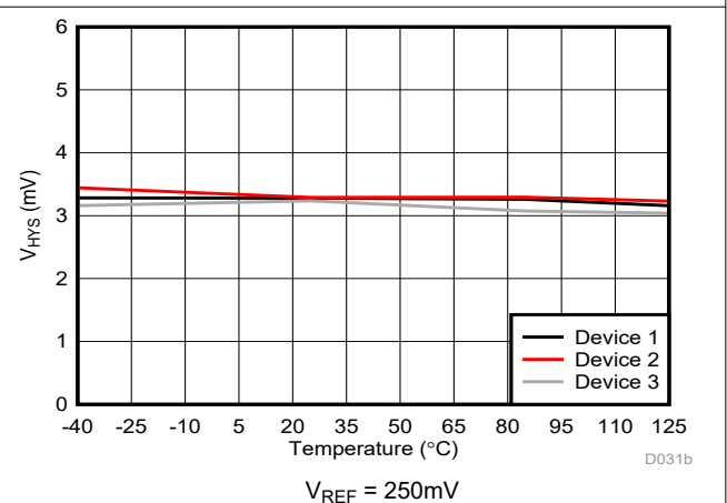
图 6-34. Cmp1 跳变阈值迟滞与温度间的关系
