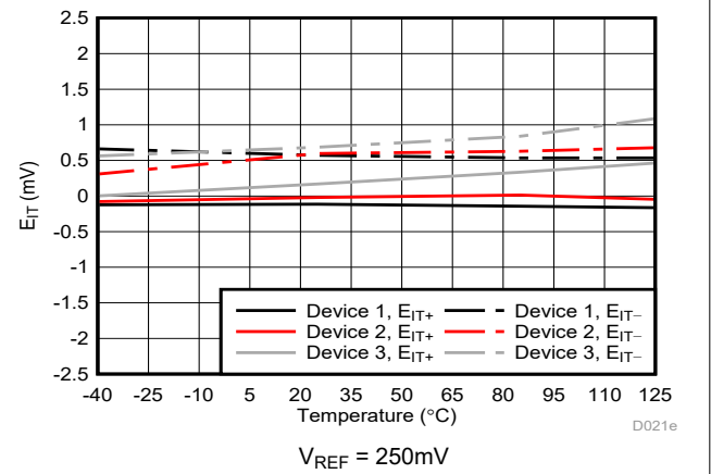
图 6-14. Cmp0 跳变阈值误差与温度间的关系
