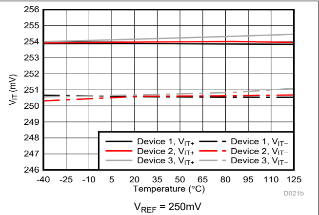
图 6-12. Cmp0 跳变阈值与温度间的关系
