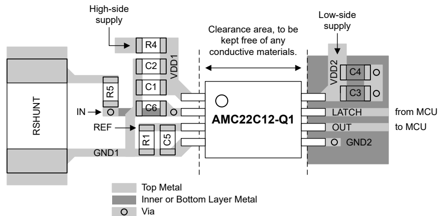
图 8-7. 建议布局 AMC22C12-Q1
