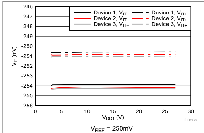
图 6-29. Cmp1 跳变阈值与电源电压间的关系
