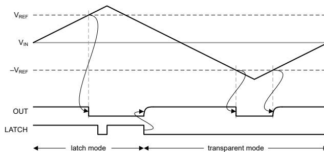
图 6-2. 功能时序图
