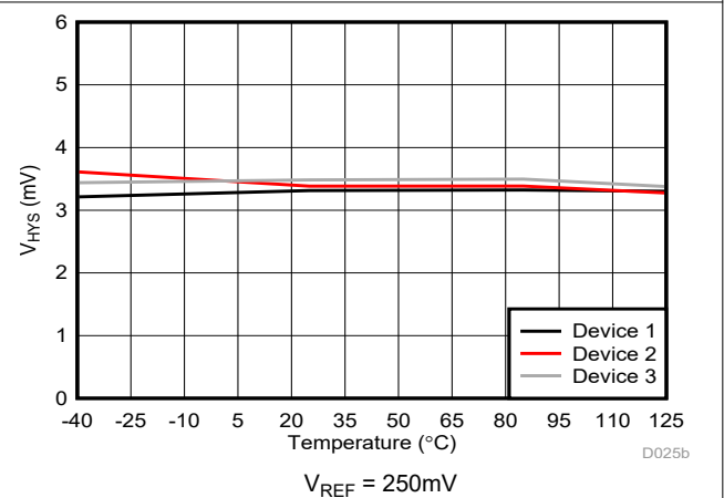
图 6-16. Cmp0 跳变阈值迟滞与温度间的关系
