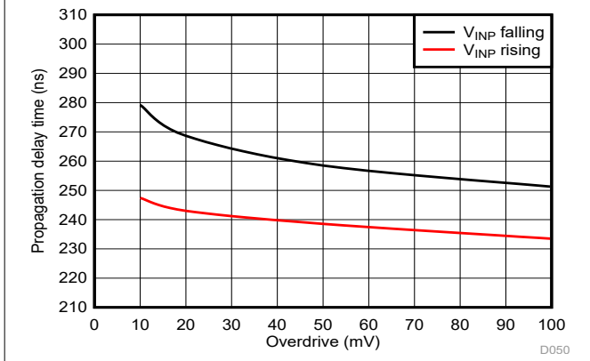
图 6-35. Cmp0 传播延迟与过驱间的关系
