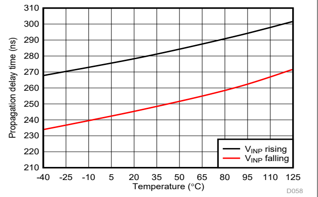
图 6-36. Cmp0 传播延迟与温度间的关系
