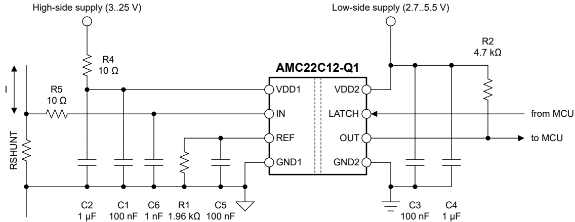
图 8-6. 去耦 AMC22C12-Q1
