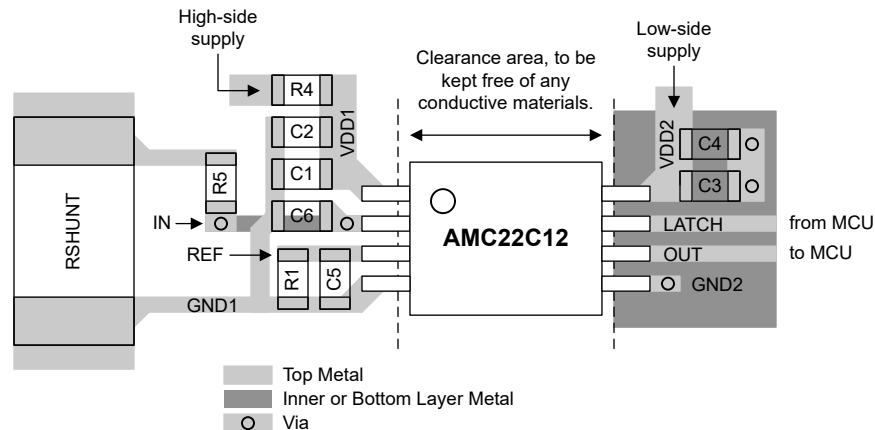
图 8-7. 建议布局 AMC22C12
