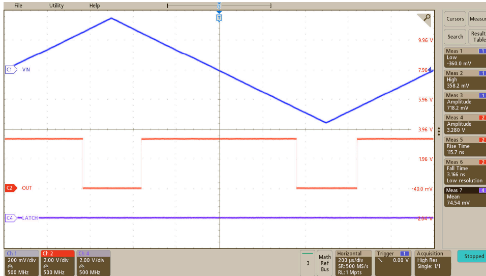
图 8-3. AMC22C12 对三角输入波形的输出响应
