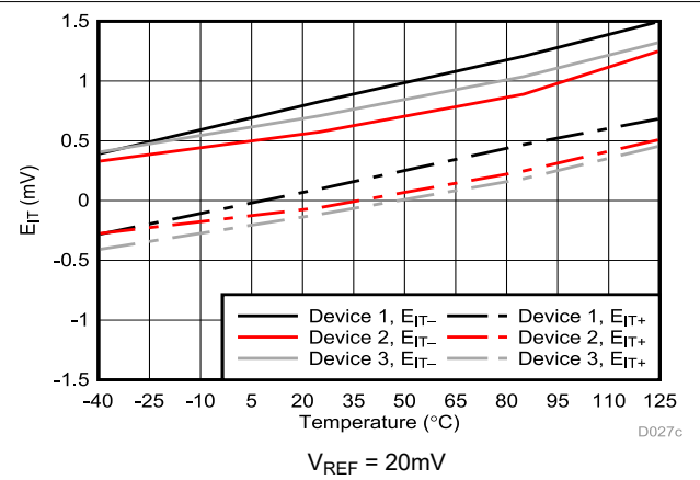
图 6-26. Cmp1 跳变阈值误差与温度间的关系
