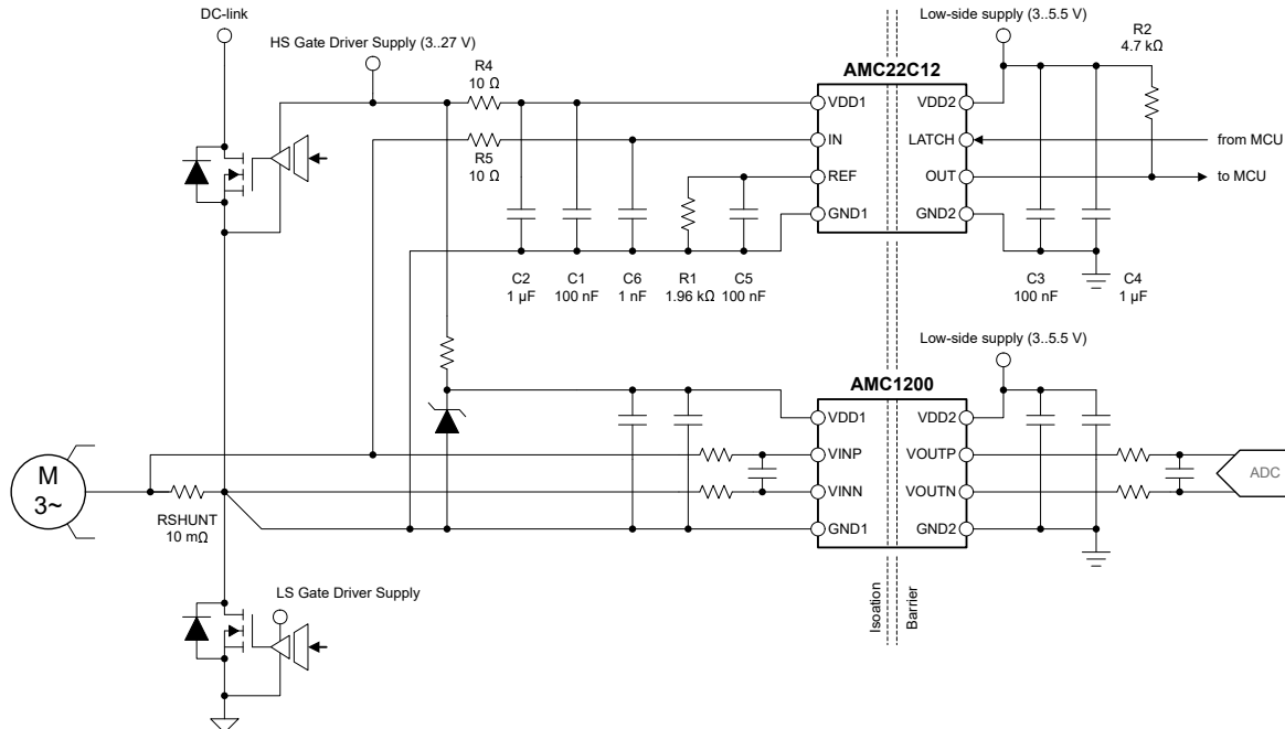
图 8-1. 使用 AMC22C12 进行过流检测
