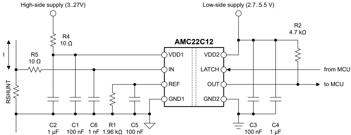
图 8-6. 去耦 AMC22C12
