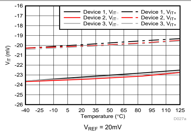
图 6-24. Cmp1 跳变阈值与温度间的关系
