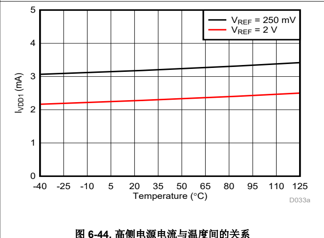
图 6-44. 高侧电源电流与温度间的关系
