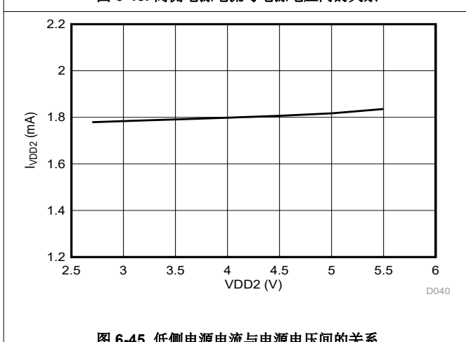
图 6-45. 低侧电源电流与电源电压间的关系
