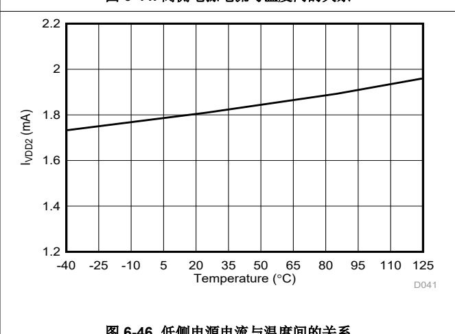
图 6-46. 低侧电源电流与温度间的关系
