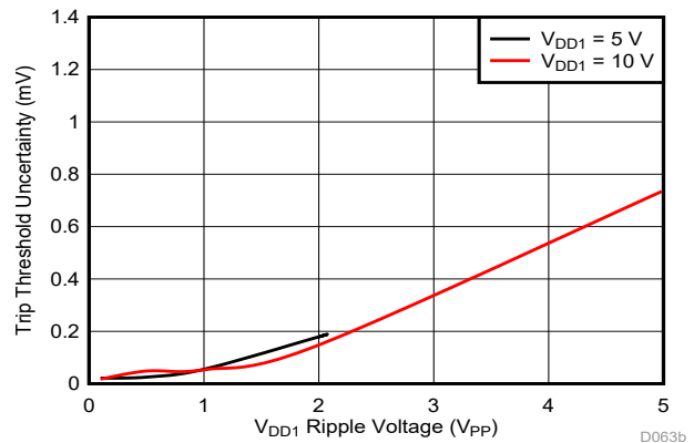
图 8-5. 跳变阈值对 V_{\text{DD1}} 纹波电压的灵敏度 ( \text{Cmp1} , f_{\text{RIPPLE}} = 10\text{kHz} )
