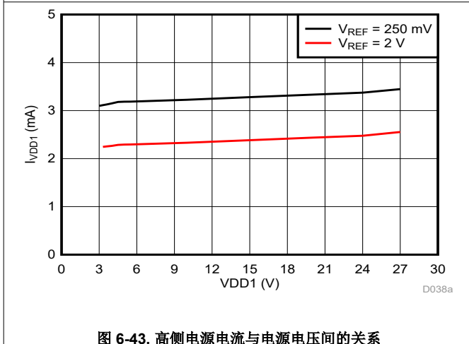
图 6-43. 高侧电源电流与电源电压间的关系
