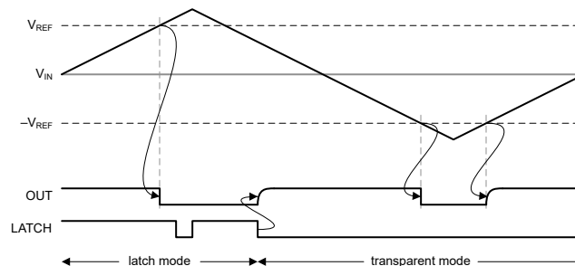
图 6-2. 功能时序图
