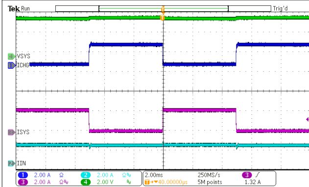
图 9-17. System Load Transient
