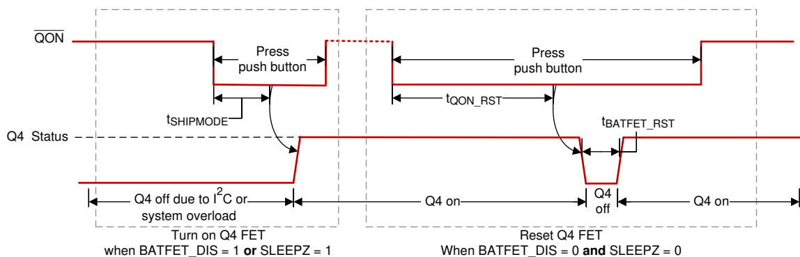
图 8-10. \overline{QON} Timing
