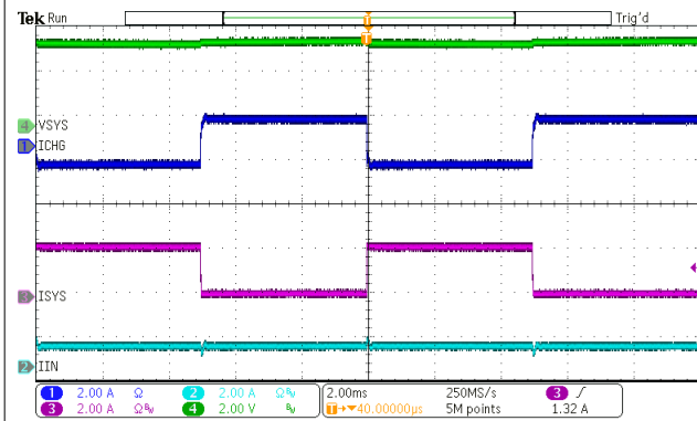
图 9-15. System Load Transient
