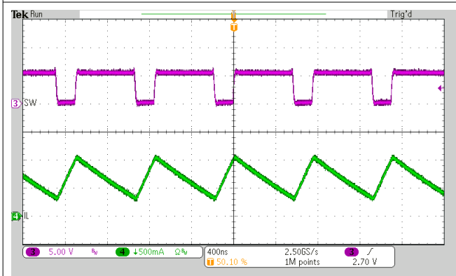
图 9-11. Charge Disable
