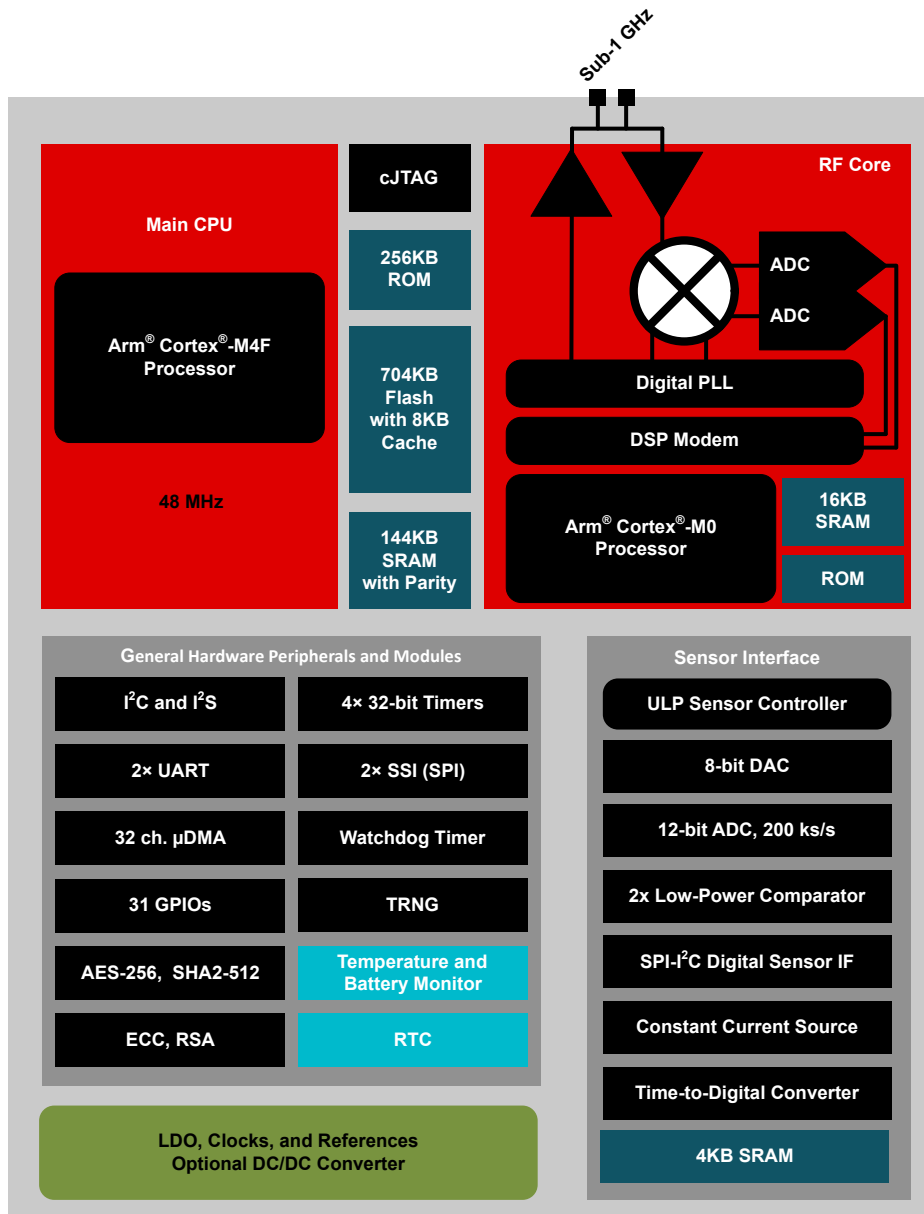
图 3-1. CC1312R7 方框图
