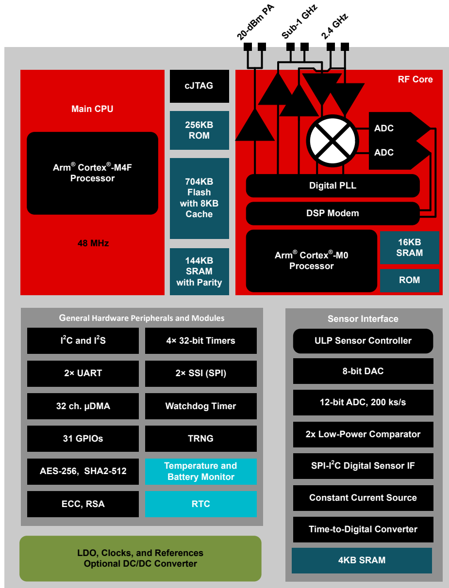
图 3-1. CC1352P7 方框图
