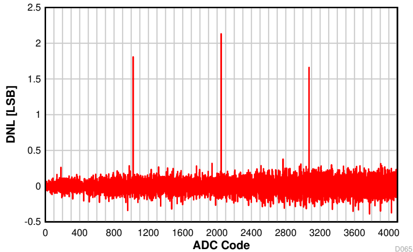
图 8-36. DNL vs. ADC Code
