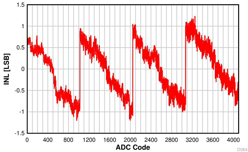
图 8-35. INL vs. ADC Code
