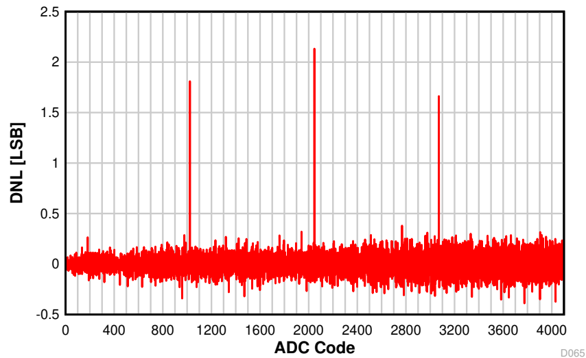
图 8-26. DNL vs. ADC Code
