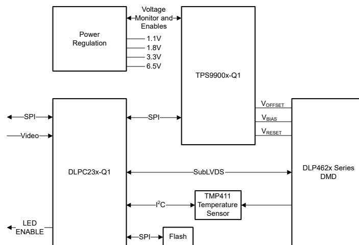
DLP4621-Q1 DLP® 芯片组系统方框图
