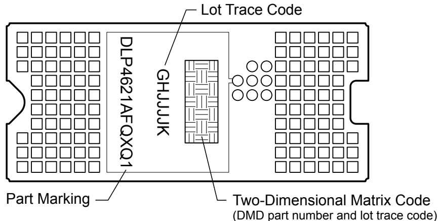
图 11-2. DMD Marking
