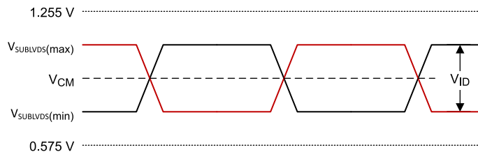
图 6-7. SubLVDS Waveform Parameters
