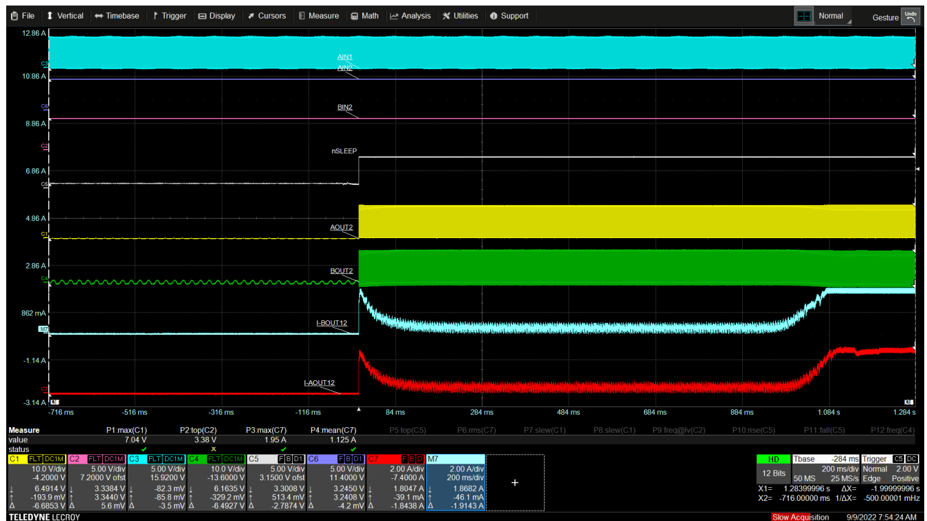
图 10-9. 无电流调节
