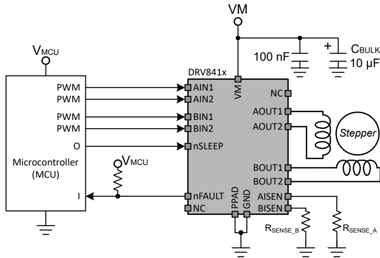
图 10-1. DRV8411 驱动步进电机的典型应用原理图
