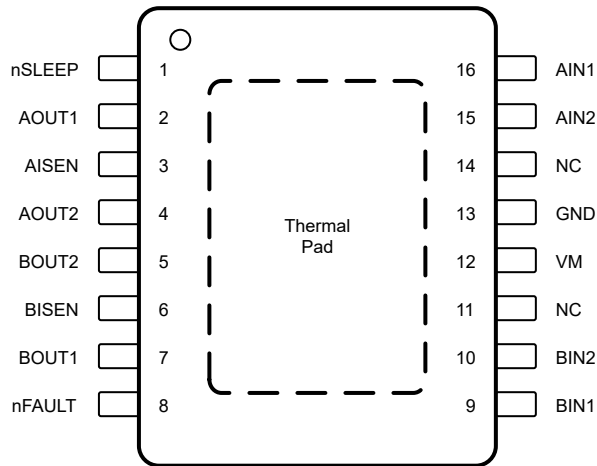
图 6-1. PWP 封装 16 引脚 HTSSOP 顶视图
