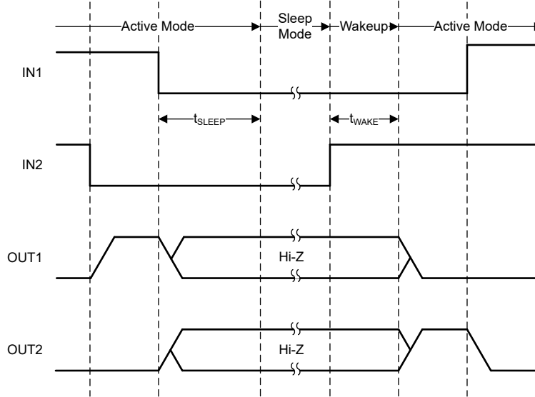
图 9-8. 睡眠模式进入和唤醒时序图
