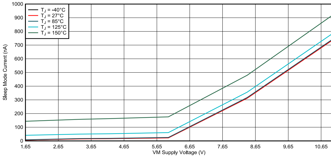
图 8-2. 睡眠模式电流
