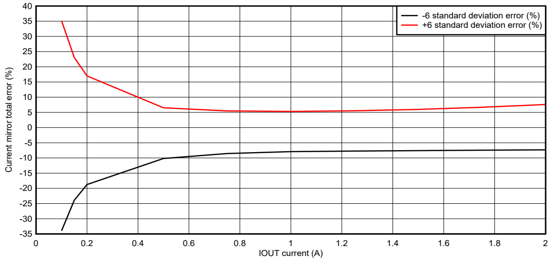
图 8-5. 电流镜比例因数，VM = 1.65V 至 3.3V
