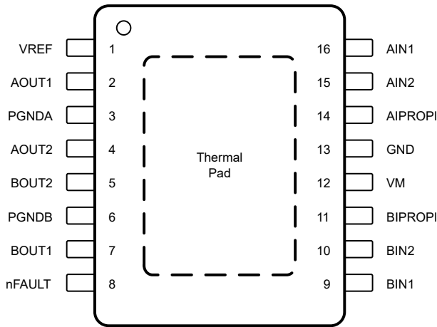
图 6-1. PWP 封装 16 引脚 HTSSOP 顶视图
