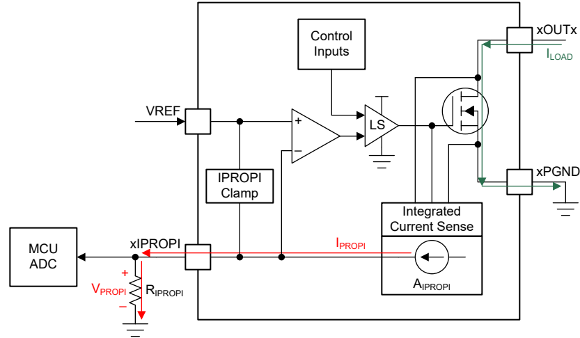
图 9-4. 集成电流感测
