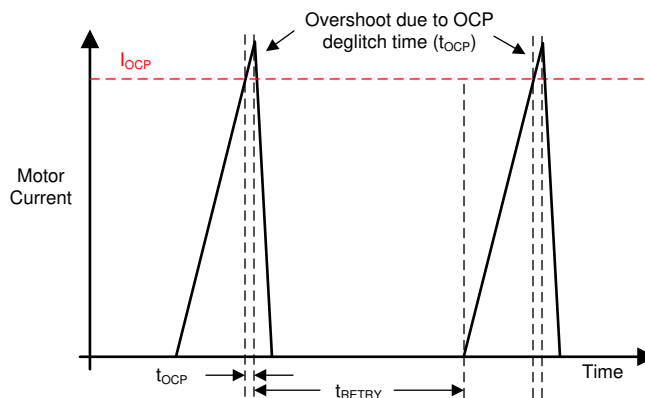
图 9-6. OCP 运行
