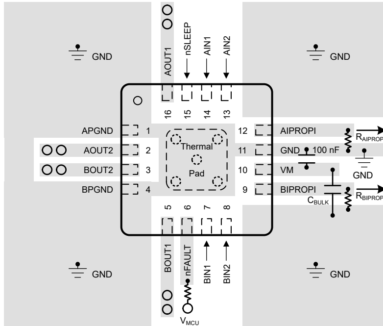
图 12-2. RTE (WQFN) 封装的建议布局示例
