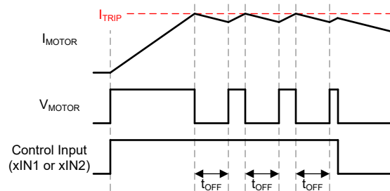
图 9-5. 关断时间电流调节
