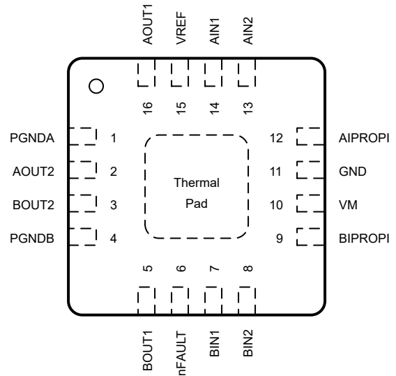
图 6-2. RTE 封装 16 引脚 WQFN 顶视图
