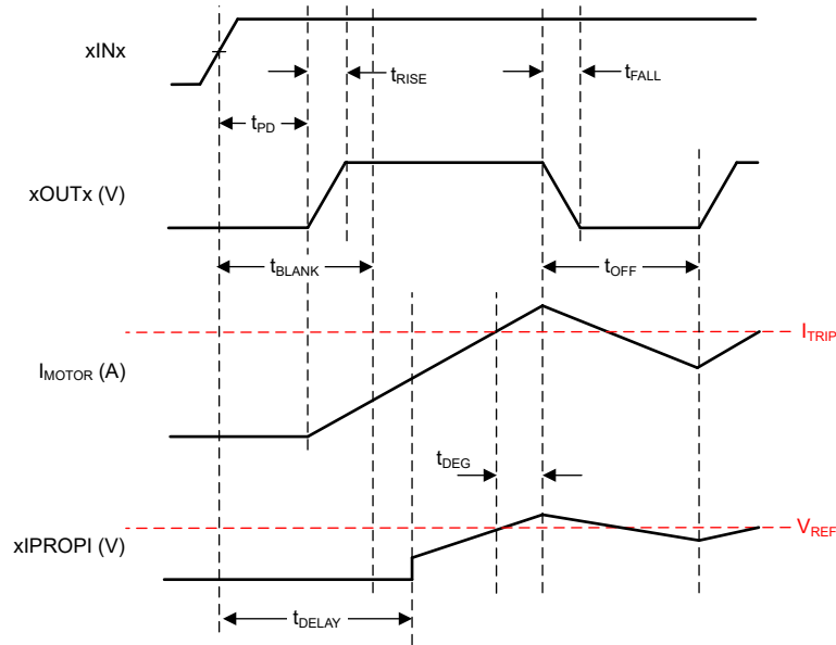
图 9-3. 详细 IPROPI 时序图
