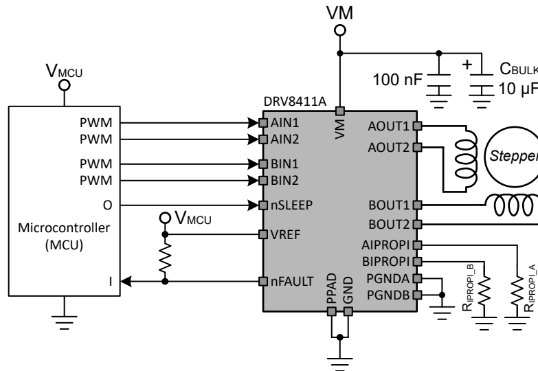
图 10-1. DRV8411A 驱动步进电机的典型应用原理图
