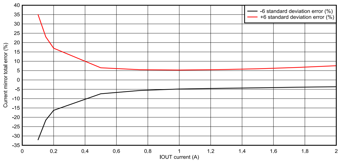
图 8-6. 电流镜比例因数，VM = 3.3V 至 11V
