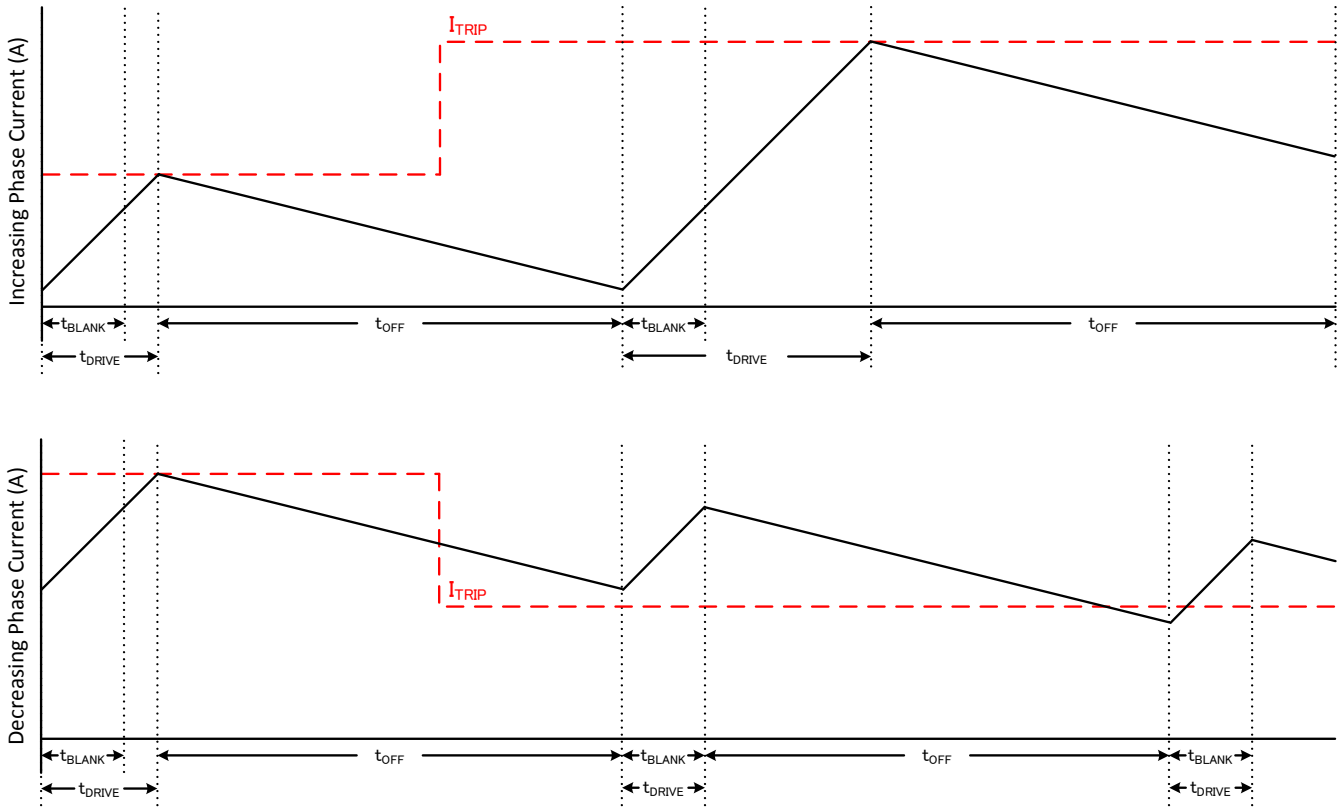
图 7-12. 慢速衰减模式
