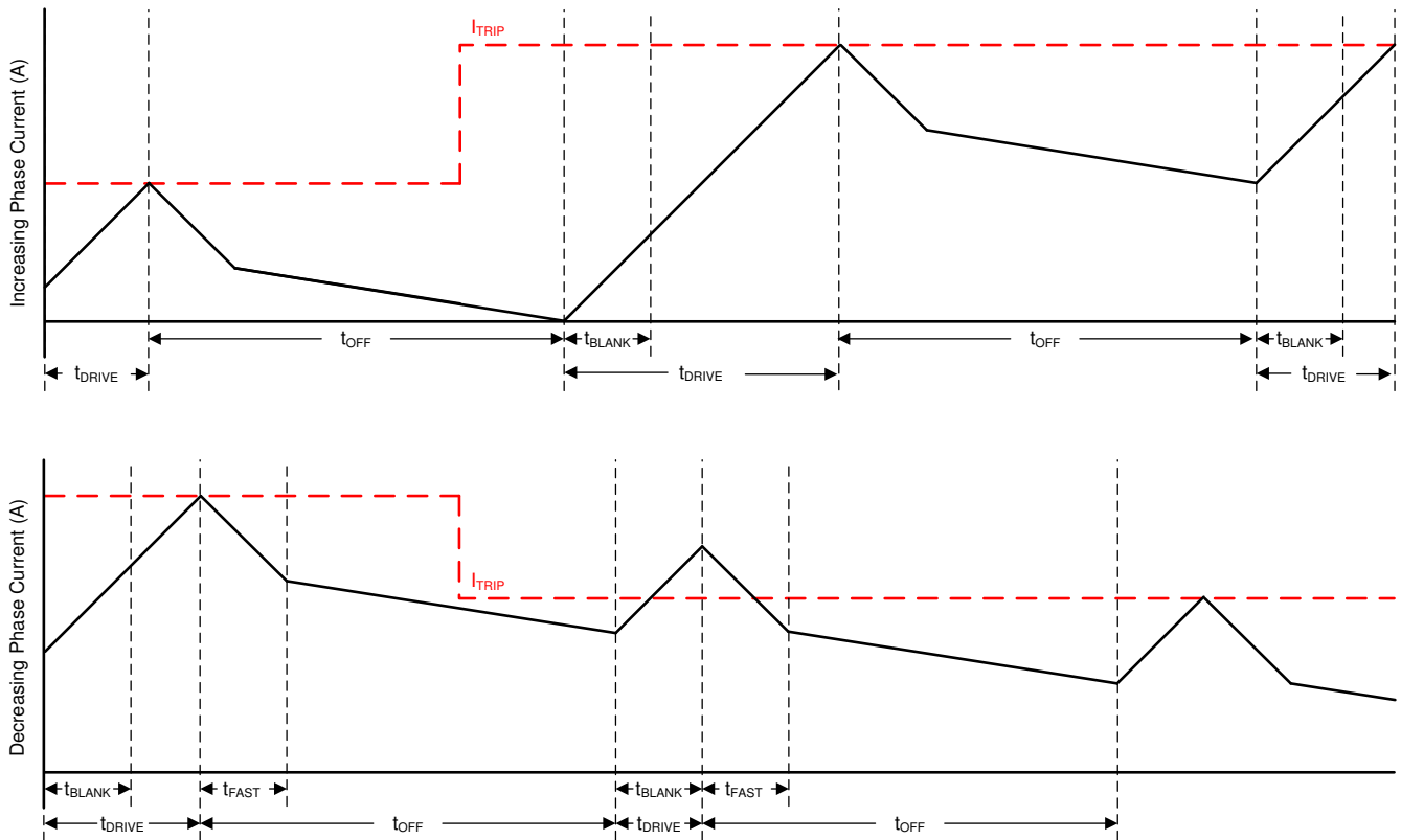
图 7-13. 混合衰减模式
