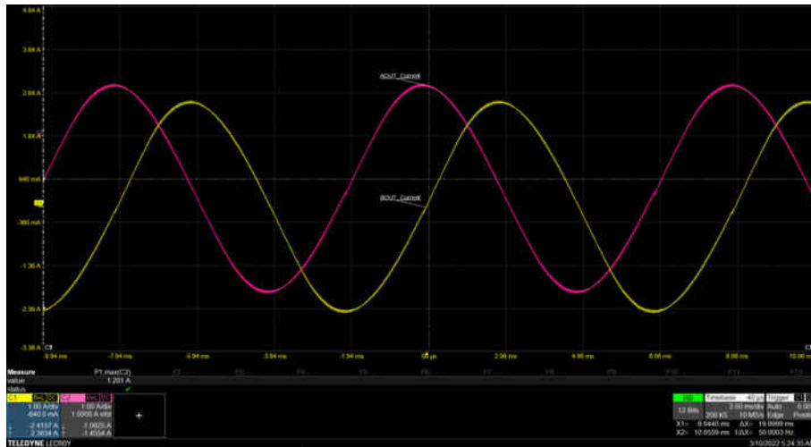
图 7-19. 静音步进衰减模式下的线圈电流波形
