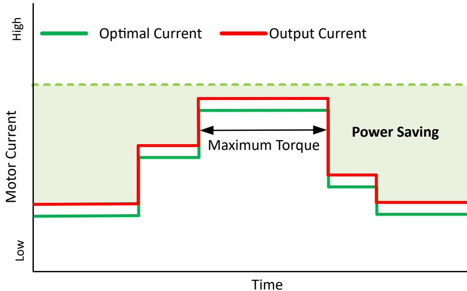
图 7-22. 通过自动扭矩实现节能
