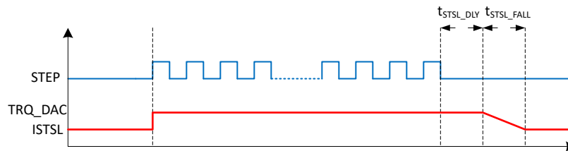
图 7-29. 静止省电模式
