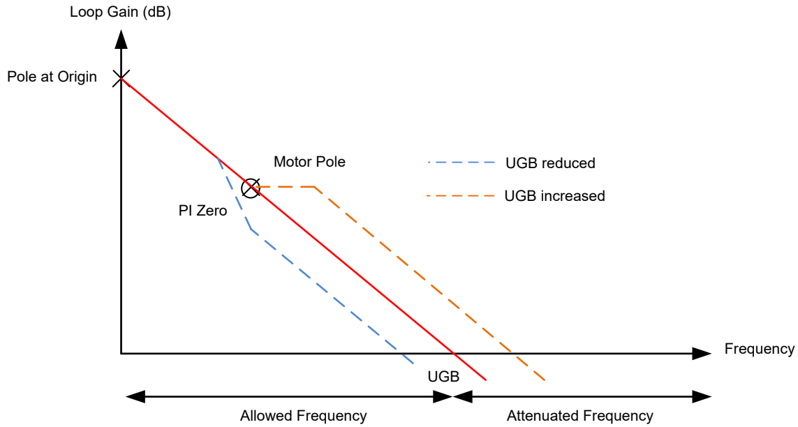
图 7-18. 静音步进增益与频率间的关系
