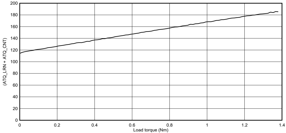
图 7-23. (ATQ_LRN + ATQ_CNT) 与负载扭矩间的关系
