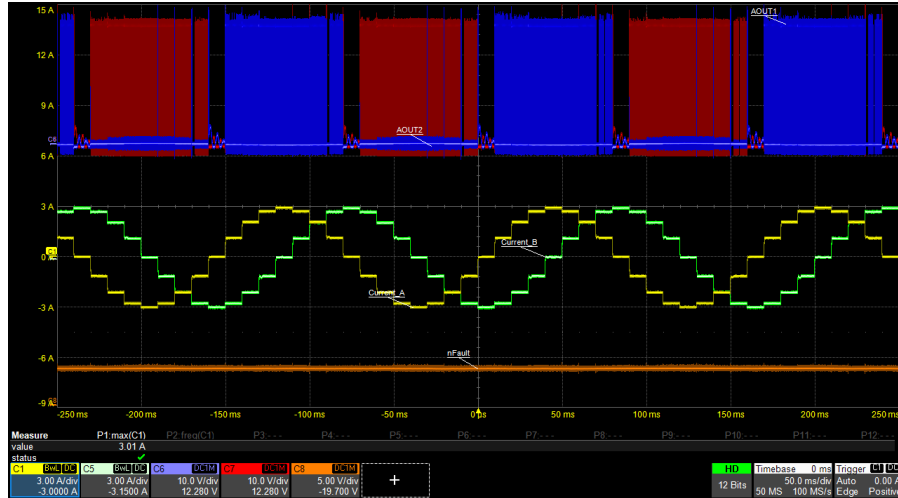
图 8-4. 在 100pps、 I_{FS} = 3A 时为 1/4 微步进
