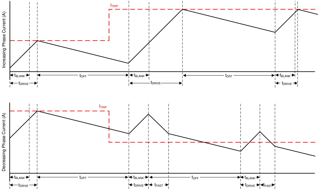
图 7-14. 智能调优动态衰减模式
