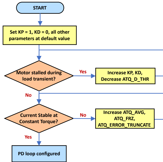
图 7-28. 选择 PD 控制环路参数
