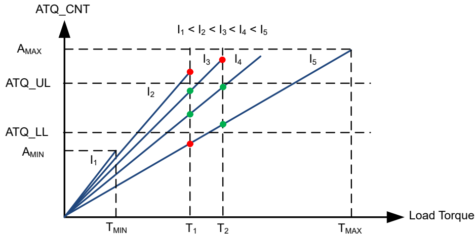
图 7-26. ATQ_CNT 作为负载转矩的函数
