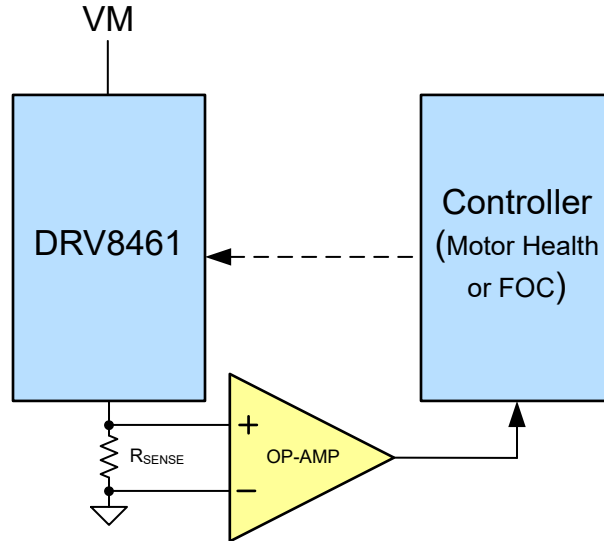
图 7-16. 使用外部电阻器进行电流检测
