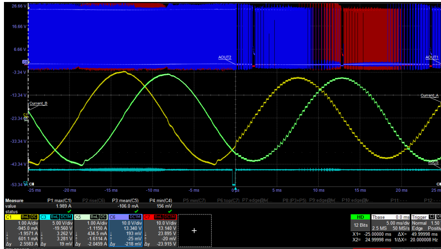
图 7-20. 静音步进至智能调优转换
