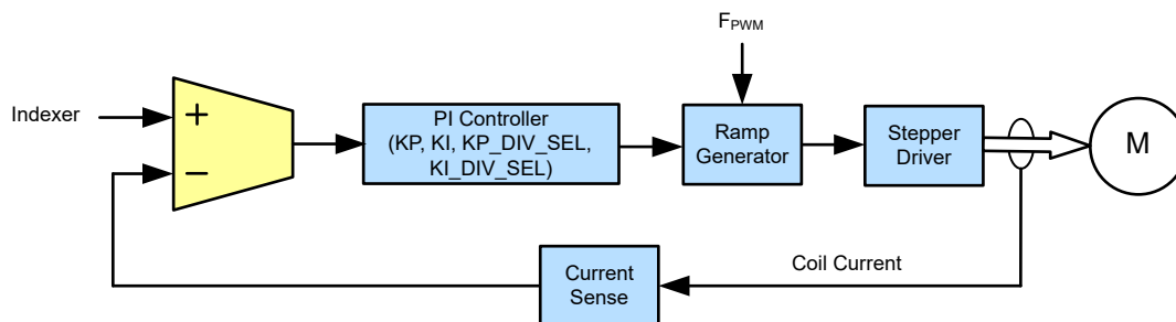
图 7-17. 静音步进方框图
