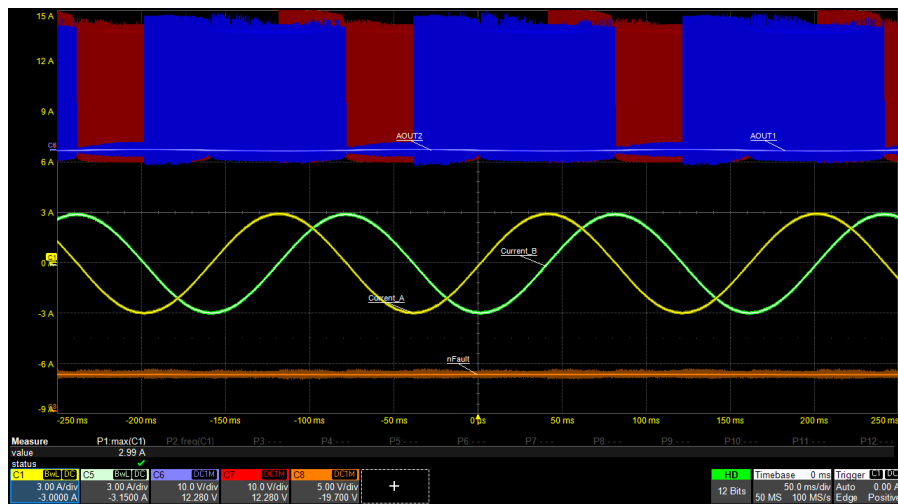
图 8-5. 在 6400pps、 I_{FS} = 3A 时为 1/256 微步进
