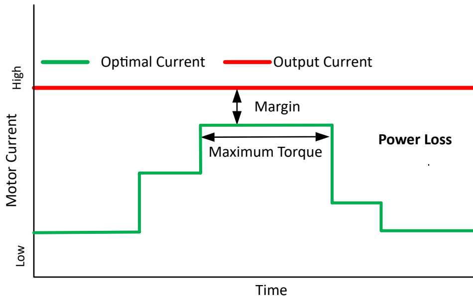
图 7-21. 传统步进电机驱动器的功率损耗
