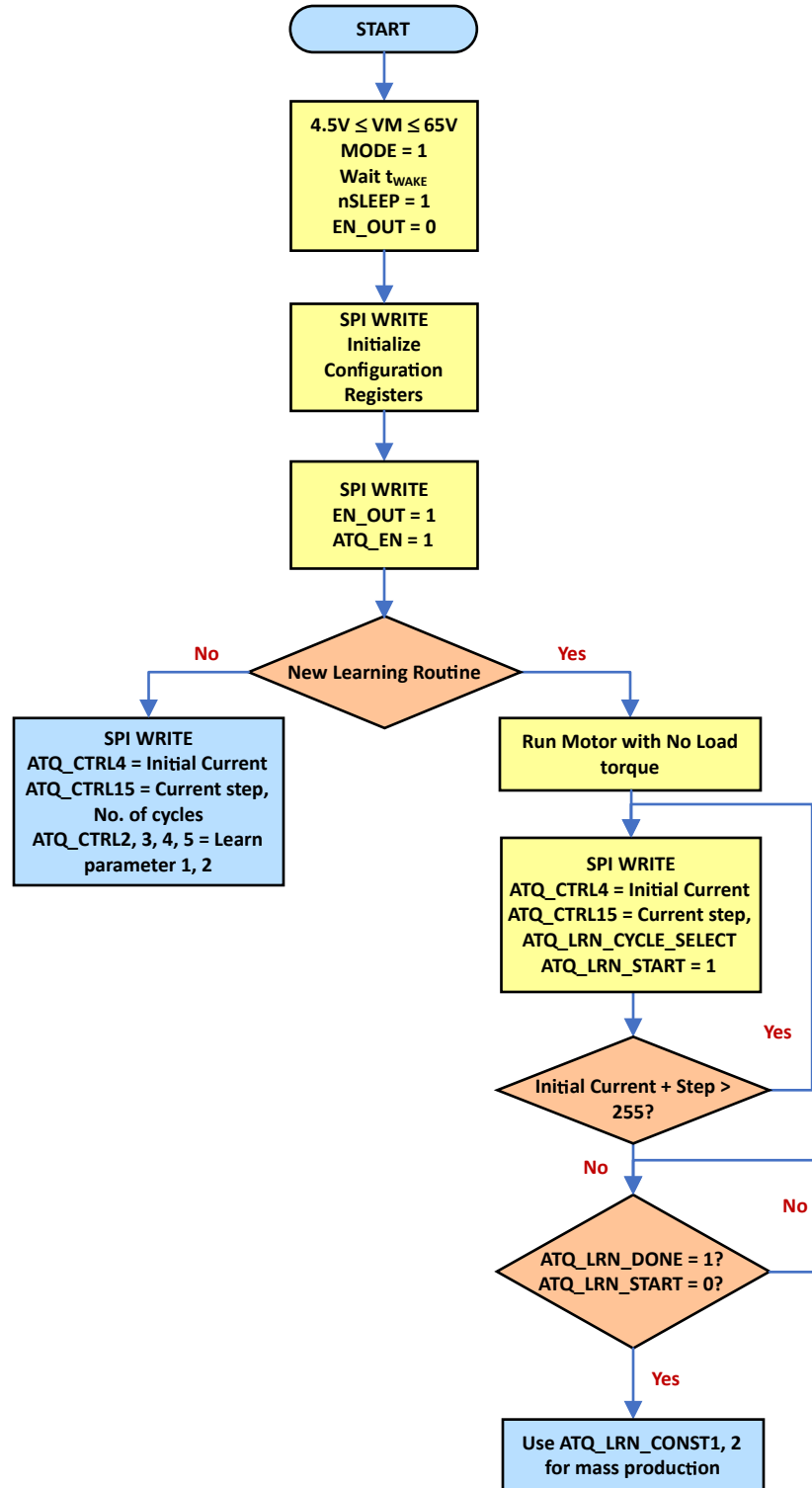
图 7-24. 自动扭矩学习流程图
