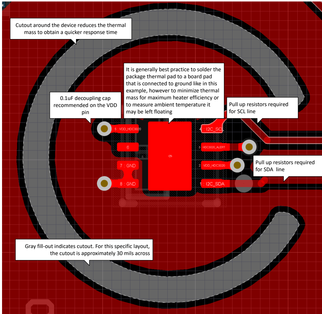
图 9-3. HDC302x-Q1 PCB 布局示例
