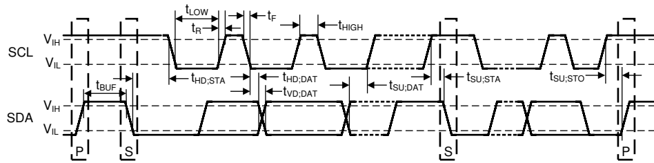
图 7-1. HDC302x-Q1 I 2 C 时序图
