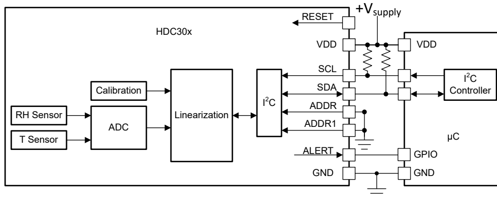
图 9-1. 典型湿度应用原理图
