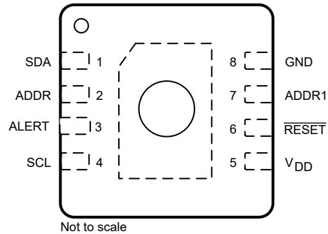
图 6-1. HDC302x-Q1 DEF、DEH、DEJ 封装 8 引脚 WSON 透明顶视图
