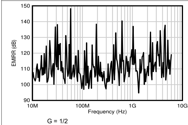
图 7-63. 差模 EMI 抑制比
