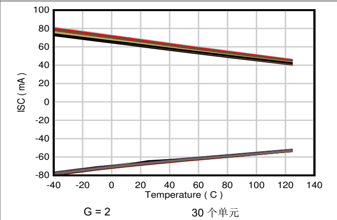
图 7-62. 短路电流与温度间的关系
