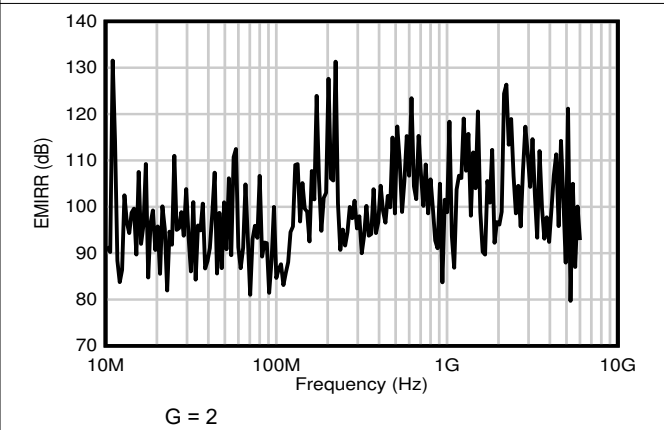
图 7-66. 共模 EMI 抑制比
