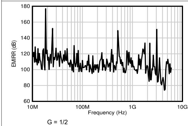
图 7-65. 共模 EMI 抑制比
