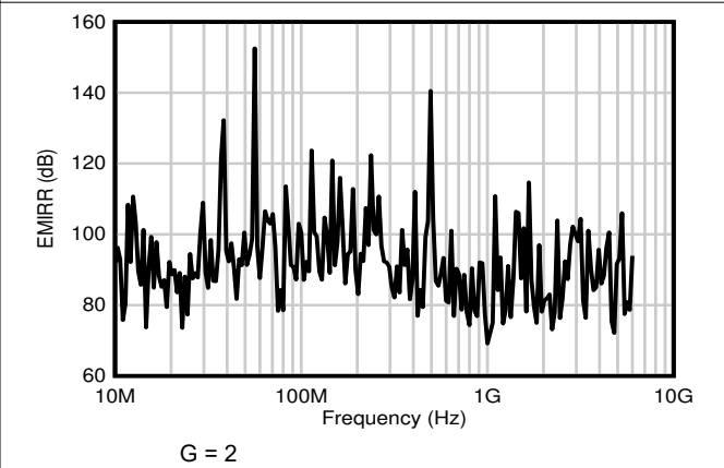
图 7-64. 差模 EMI 抑制比
