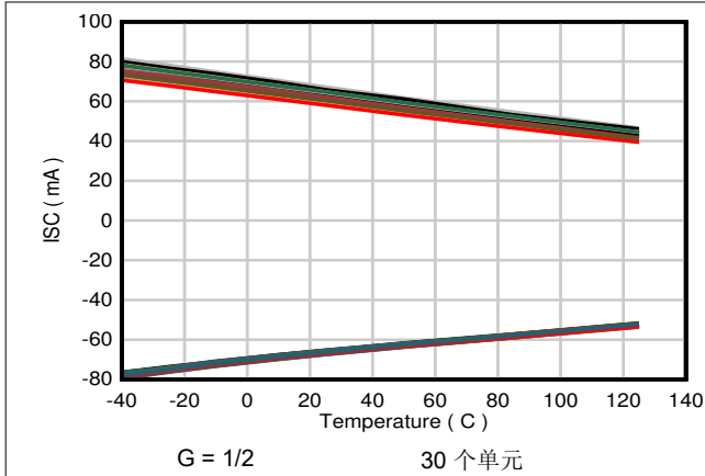
图 7-61. 短路电流与温度间的关系
