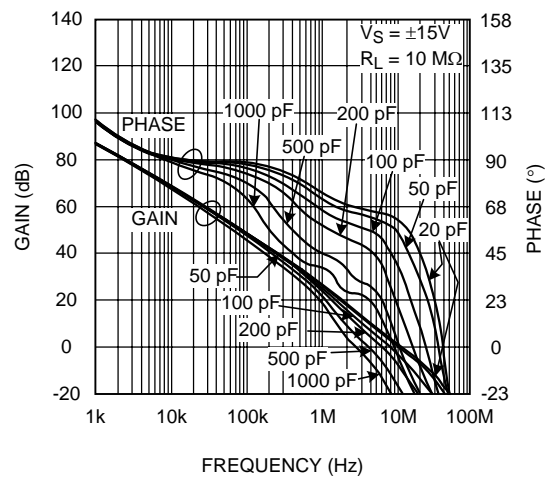
图 42. 各种容性负载下的开环频率响应
