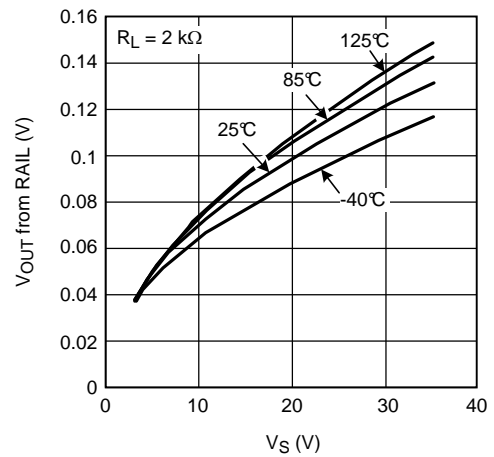
图 40. 负输出摆幅与电源电压间的关系
