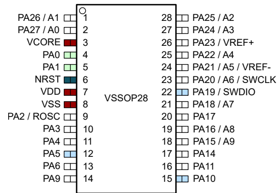
图 6-3. 28 引脚 DGS28 (VSSOP) (俯视图) - MSPM0L130x
