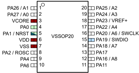
图 6-6. 20 引脚 DGS20 (VSSOP) (俯视图) - MSPM0L130x
