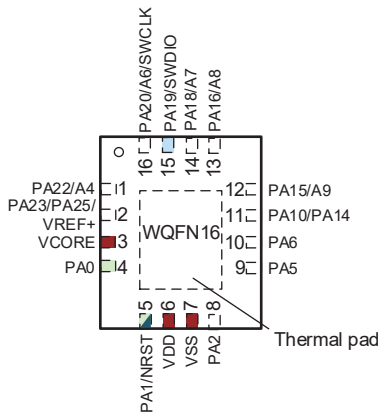
图 6-8. 16 引脚 RTR (WQFN) (俯视图) - MSPM0L130x
