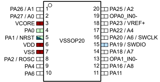
图 6-7. 20 引脚 DGS20 (VSSOP) (俯视图) - MSPM0L134x
