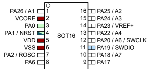
图 6-9. 16 引脚 DYY (SOT) (俯视图) - MSPM0L130x
