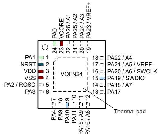
图 6-5. 24 引脚 RGE (VQFN) (俯视图) - MSPM0L130x
