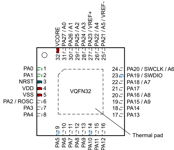
图 6-2. 32 引脚 RHB (VQFN) (俯视图) - MSPM0L130x
