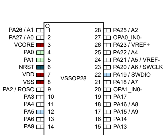
图 6-4. 28 引脚 DGS28 (VSSOP) (俯视图) - MSPM0L134x
