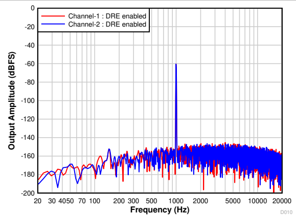
图 7-10. PCM1820-Q1: FFT With a -60-dBr Input and DRE Enabled
