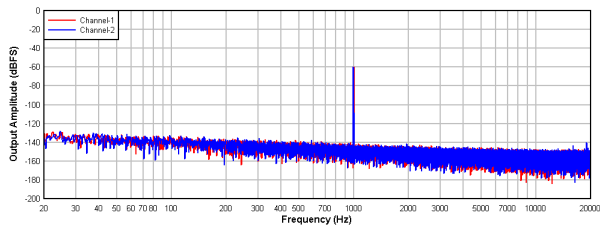
图 9-6. PCM1821-Q1: FFT With a -60-dBr Input
