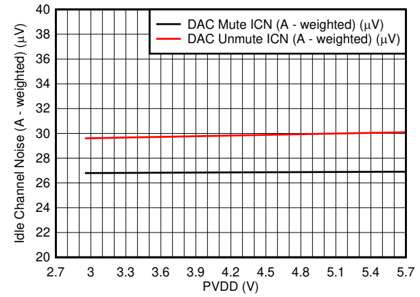
图 6-16. ICN (A-Weighted) vs PVDD
