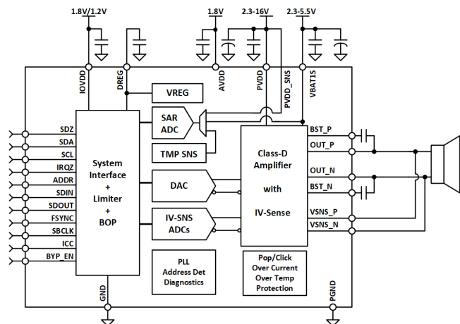
原理图
