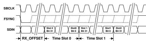
图 8-3. TDM RX Time Slots
