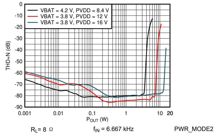
图 6-10. THD+N vs Output Power
