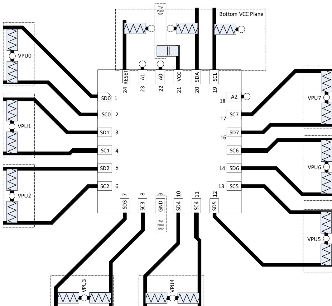
图 9-1. Layout Schematic
