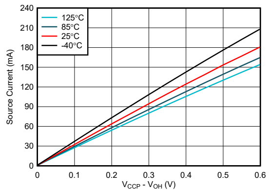
图 6-18. I/O 拉电流与输出高电压的关系， V CCP = 3.6V
