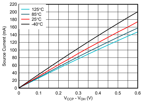
图 6-17. I/O 拉电流与输出高电压的关系， V CCP = 3.3V
