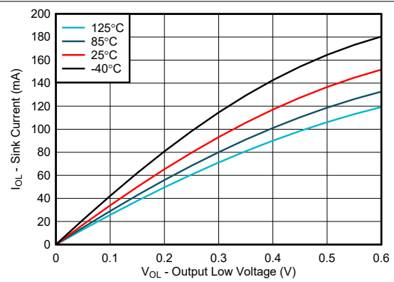
图 6-8. I/O 灌电流与输出低电压的关系, V_{CCP} = 1.8\text{V}
