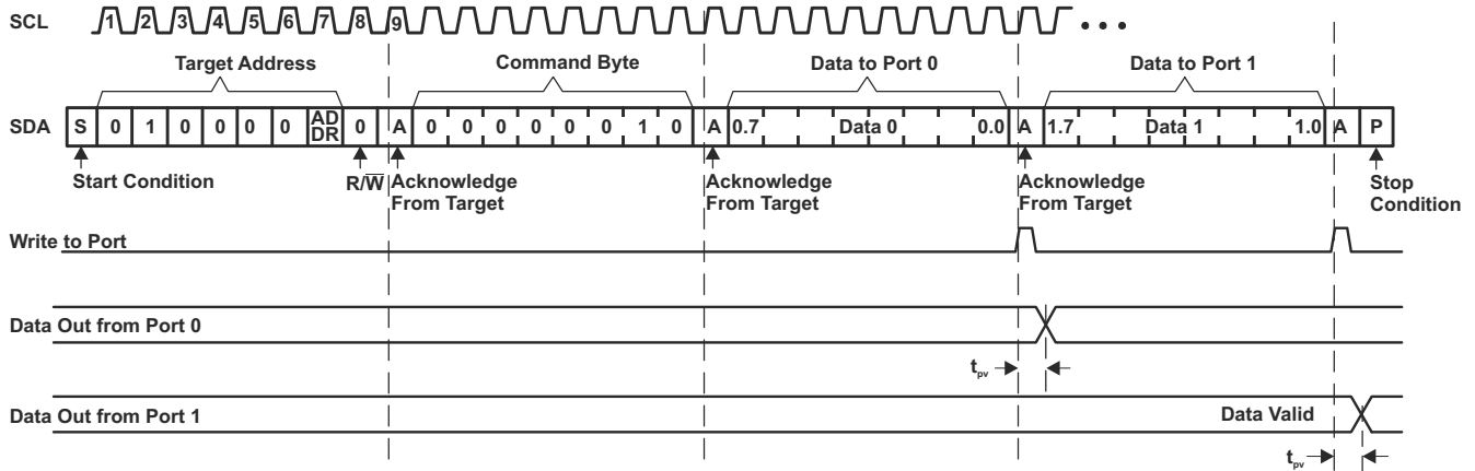
图 8-9. 对输出端口寄存器进行写入
