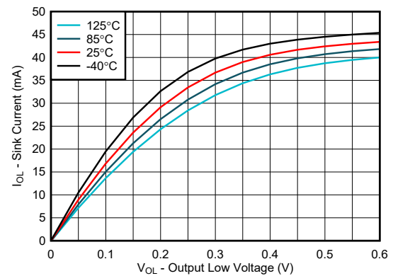
图 6-6. I/O 灌电流与输出低电压的关系, V_{CCP} = 1.08\text{V}
