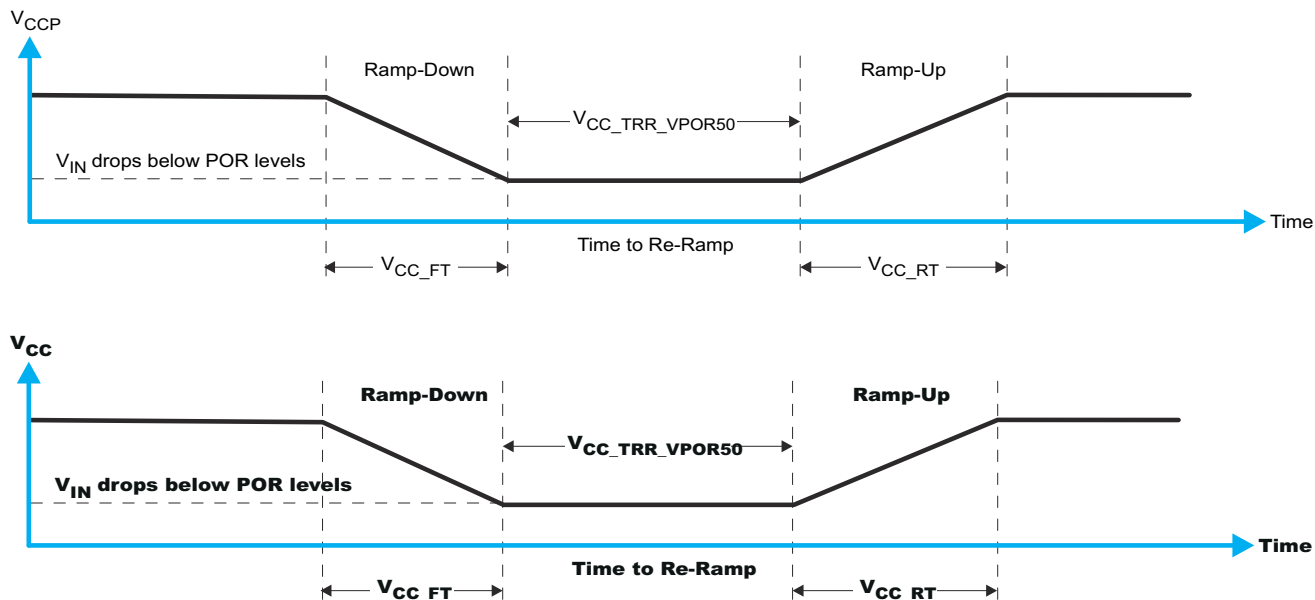
图 9-7. 将 V_{CCP} 降至低于 POR 阈值，然后重新上升
