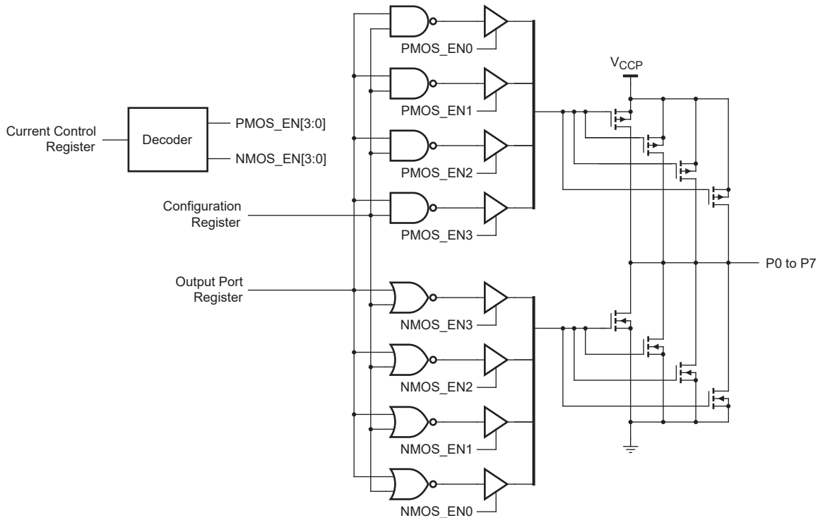
图 8-3. 简化的输出级
