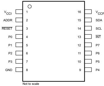
图 5-1. PW (TSSOP) 封装，16 引脚 (俯视图)
