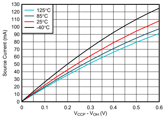
图 6-15. I/O 拉电流与输出高电压的关系， V CCP = 1.8V
