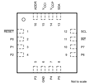
图 5-2. RSV (UQFN) 封装，16 引脚 (俯视图)
