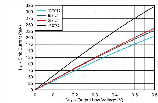
图 6-11. I/O 灌电流与输出低电压的关系, V_{CCP} = 3.6\text{V}
