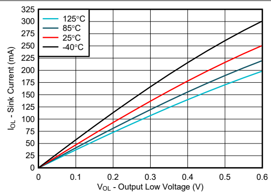
图 6-10. I/O 灌电流与输出低电压的关系, V_{CCP} = 3.3\text{V}
