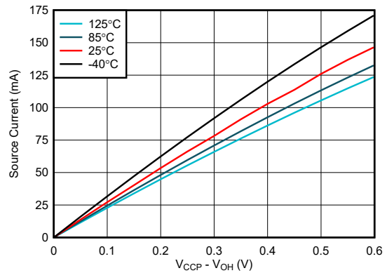
图 6-16. I/O 拉电流与输出高电压的关系， V CCP = 2.5V
