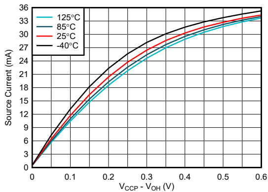
图 6-13. I/O 拉电流与输出高电压的关系， V CCP = 1.08V
