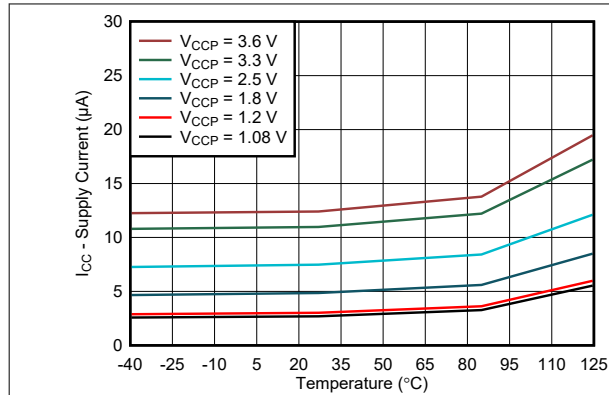
图 6-1. 电源电流与温度间的关系 - FM 模式
