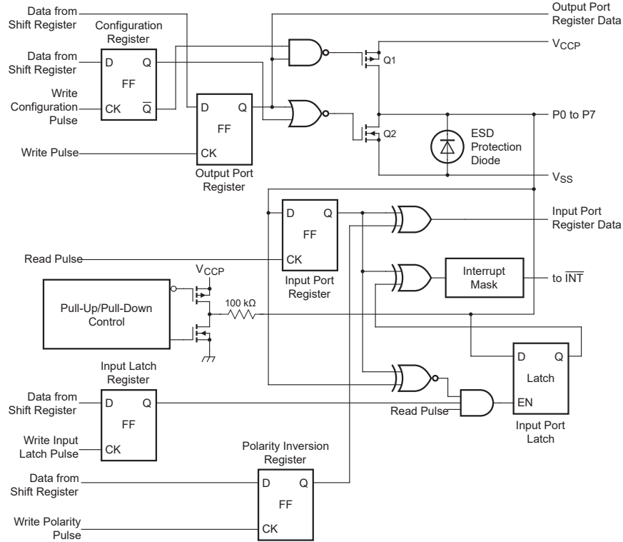
图 8-2. P0 至 P7 的简化原理图
