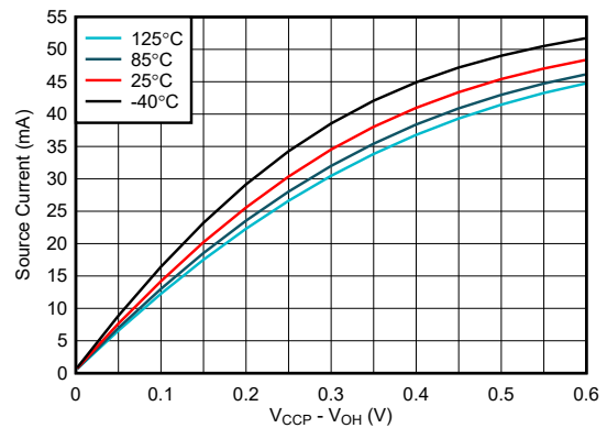
图 6-14. I/O 拉电流与输出高电压的关系， V CCP = 1.2V
