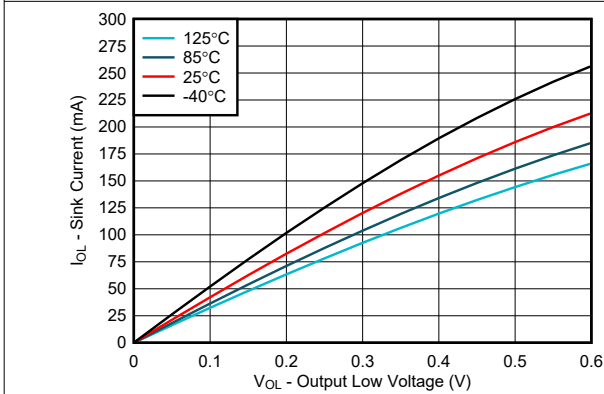
图 6-9. I/O 灌电流与输出低电压的关系, V_{CCP} = 2.5\text{V}
