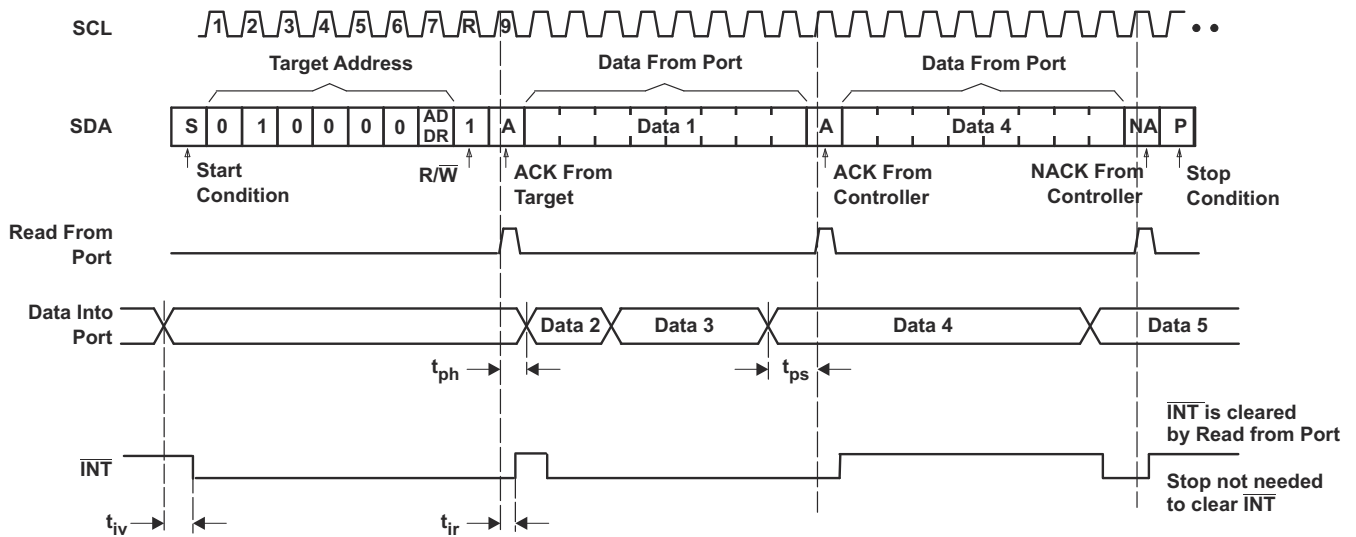
图 8-11. 从寄存器读取
