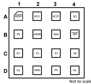
图 5-3. DTU (X2QFN) 封装，16 引脚 (俯视图)
