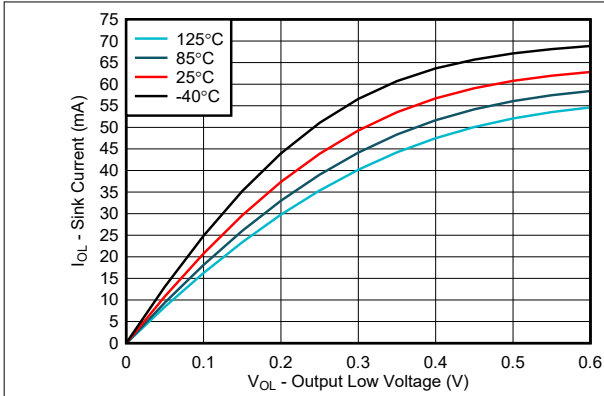
图 6-7. I/O 灌电流与输出低电压的关系, V_{CCP} = 1.2\text{V}
