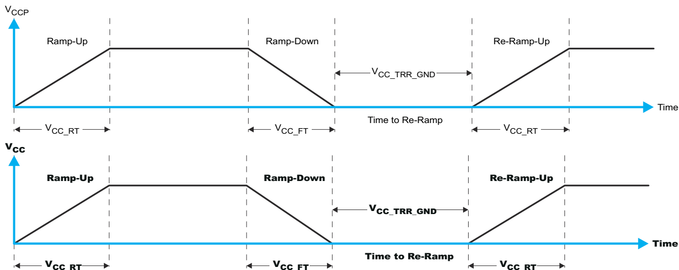
图 9-6. 将 V_{CCP} 降至 0.2V 或 0V 以下，然后上升
