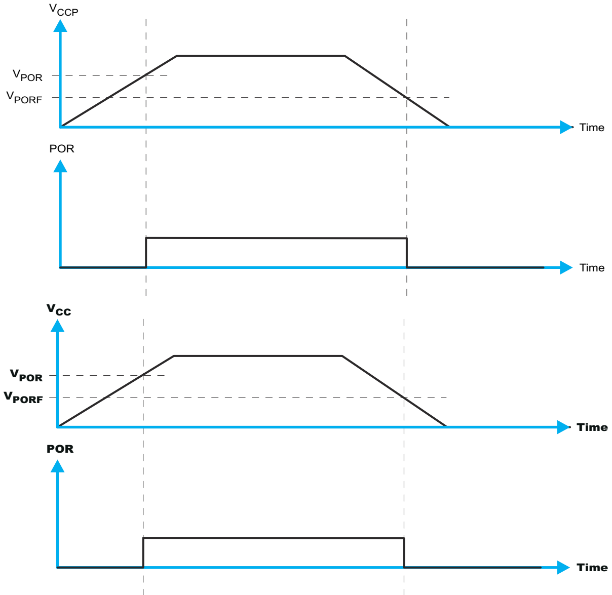
图 9-9. V POR
