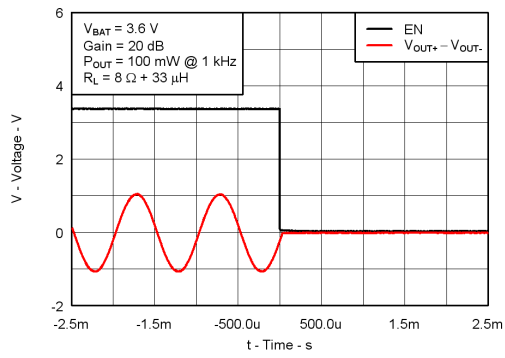
图 30. Shutdown Timing
