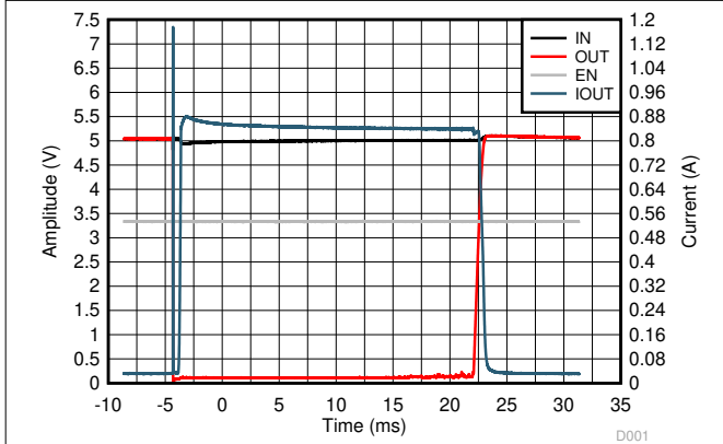
图 6-3. Pulsed Output Short
