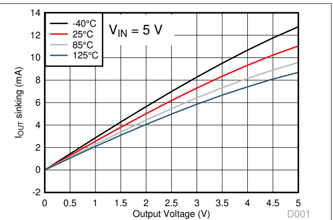
图 6-6. Output Discharge Current vs Output Voltage
