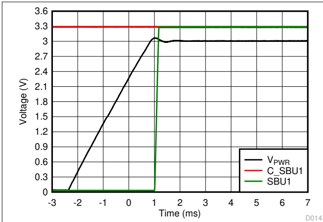
图 7-13. SBU FET Turnon Timing
