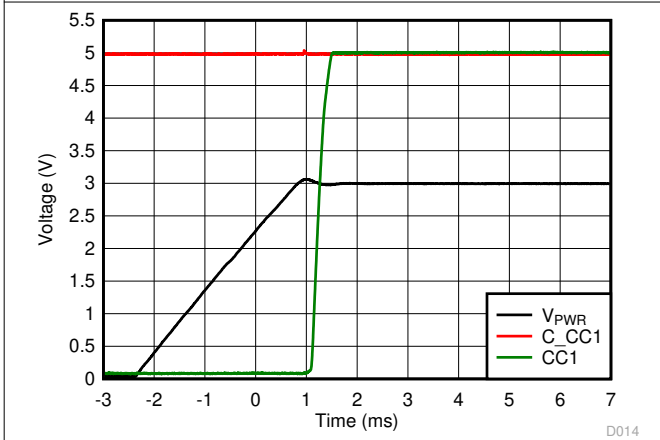
图 7-27. CC FET Turnon Timing
