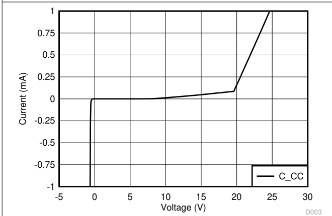
图 7-29. C CC IV Curve
