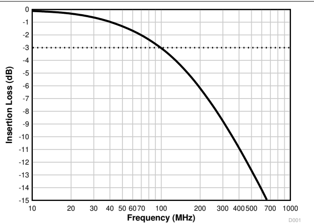
图 7-16. CC Bandwidth
