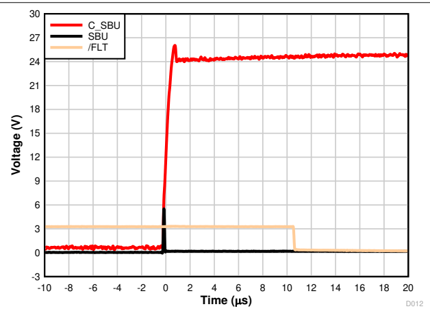
图 7-4. SBU Short-to- V_{BUS} 24 V Zoomed Out
