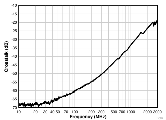
图 7-2. SBU Crosstalk
