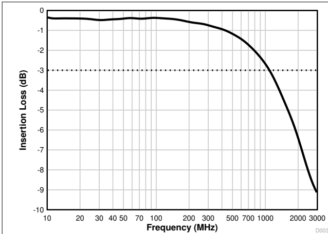
图 7-1. SBU Bandwidth
