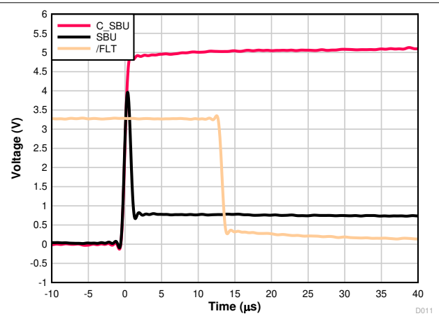
图 7-6. SBU Short-to- V_{BUS} 5 V Zoomed Out
