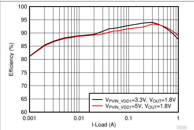
图 8-4. VDD1 Efficiency Curve, V_{OUT} = 1.8\text{ V}
