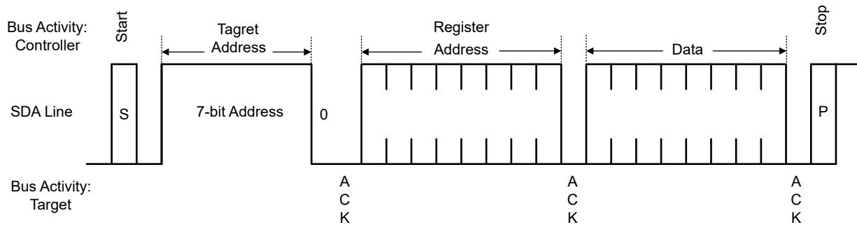
图 7-11. I 2 C Bus Write
