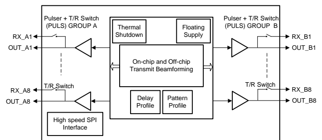
简化方框图
