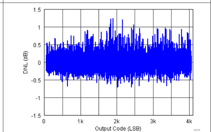
图 7-25. DNL
