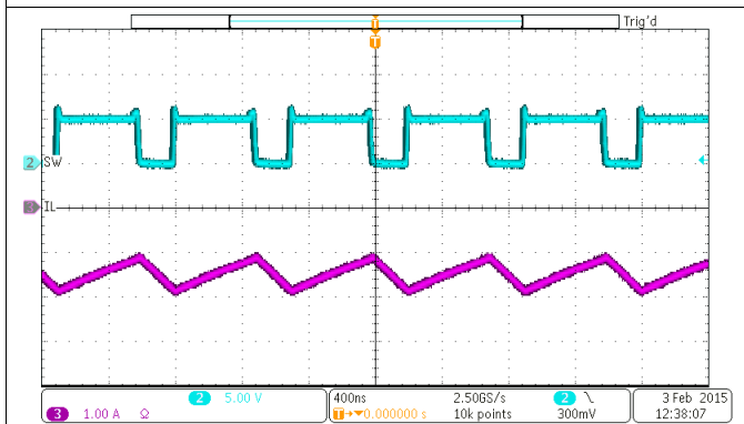
图 53. PWM Switching Waveform
