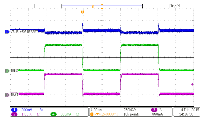
图 54. PFM Switching Waveform
