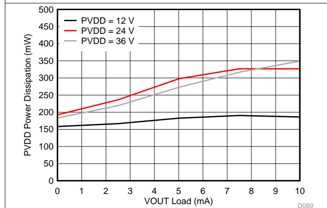
图 90. VOUT Power Dissipation vs Load
