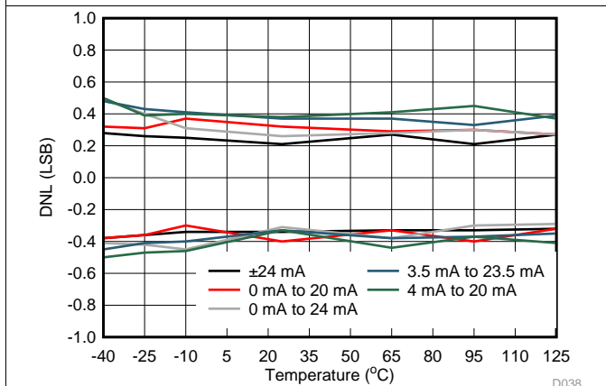
图 42. IOUT DNL vs Temperature
