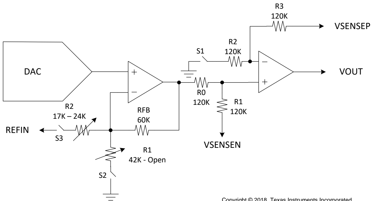
图 98. Voltage Output
