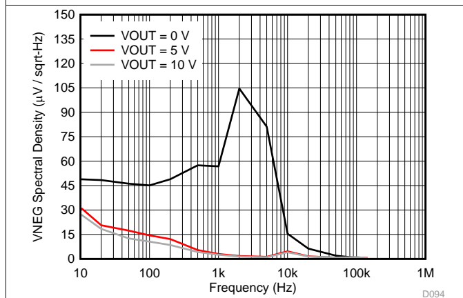
图 94. VPOS VNEG Noise Spectral Density
