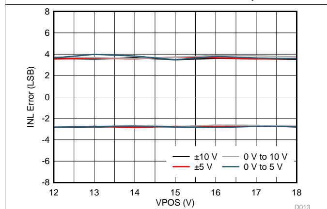
图 17. VOUT INL vs VPOS
