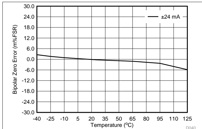
图 44. IOOUT Bipolar Zero Error vs Temperature
