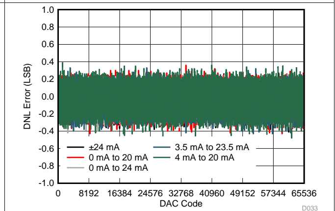
图 35. IOUT DNL vs Code (DC/DC Enabled)
