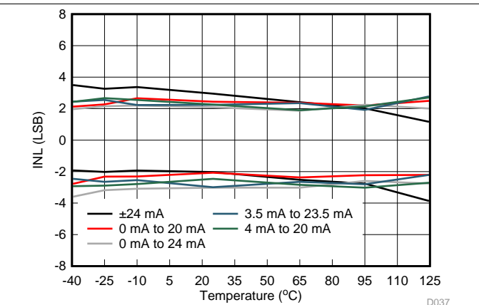
图 41. IOUT INL vs Temperature
