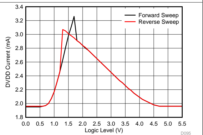
图 95. DVDD Iq vs Logic Level
