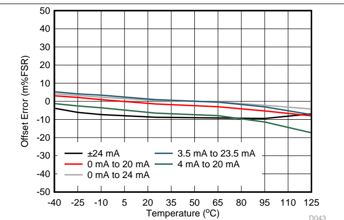
图 47. IOOUT Offset Error vs Temperature
