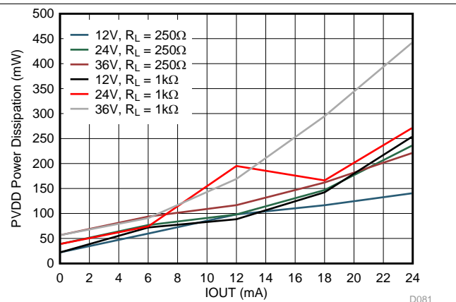
图 83. IOUT Power Dissipation vs Load
