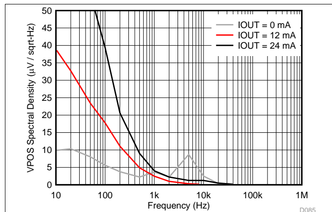
图 86. IOUT VPOS Noise Spectral Density
