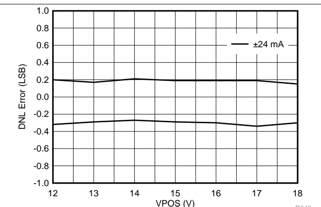
图 51. IOUT Bipolar Range DNL vs VPOS
