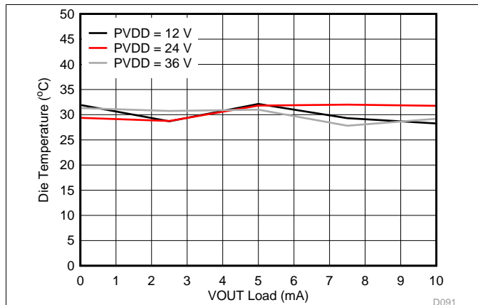
图 92. VOUT Die Temperature vs Load
