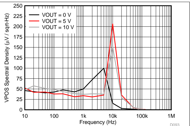
图 93. VOUT VPOS Noise Spectral Density
