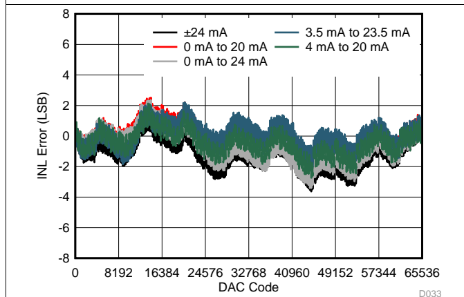
图 36. IOUT INL vs Code (DC/DC Enabled)
