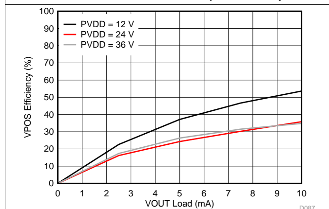
图 88. VOUT VPOS Efficiency vs Load
