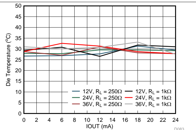
图 85. IOUT Die Temperature vs Load
