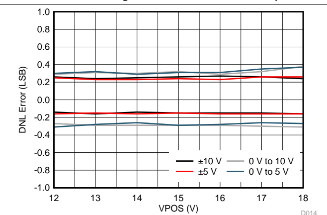
图 18. VOUT DNL vs VPOS
