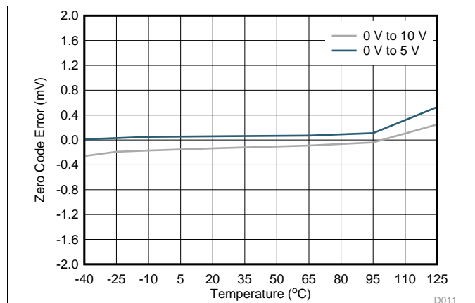
图 15. VOUT Zero-Code Error vs Temperature
