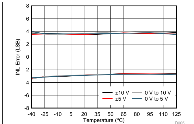
图 9. VOUT INL vs Temperature
