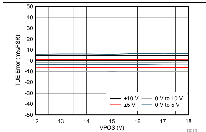
图 19. VOUT TUE vs VPOS
