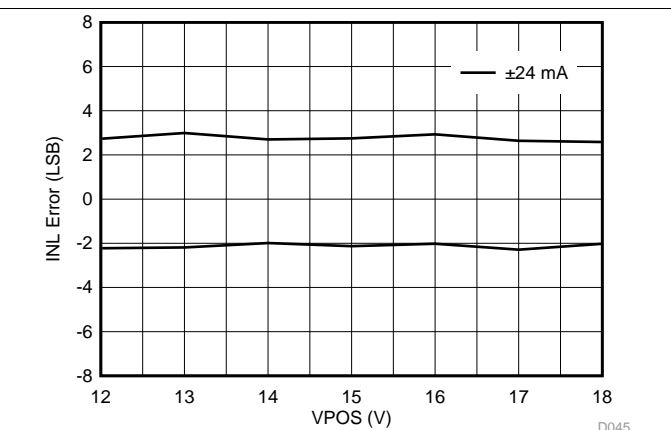
图 49. IOOUT Bipolar Range INL vs VPOS
