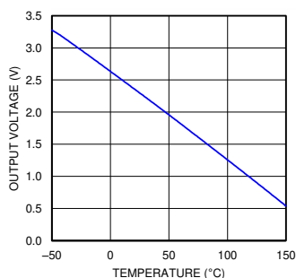
图 9-2. 模拟输出传递函数
