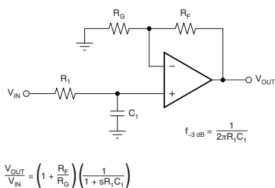
单极低通滤波器
