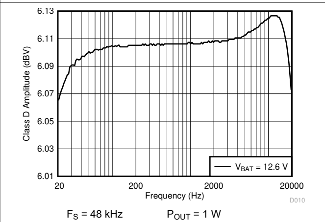
图 6-10. Amplitude vs Frequency
